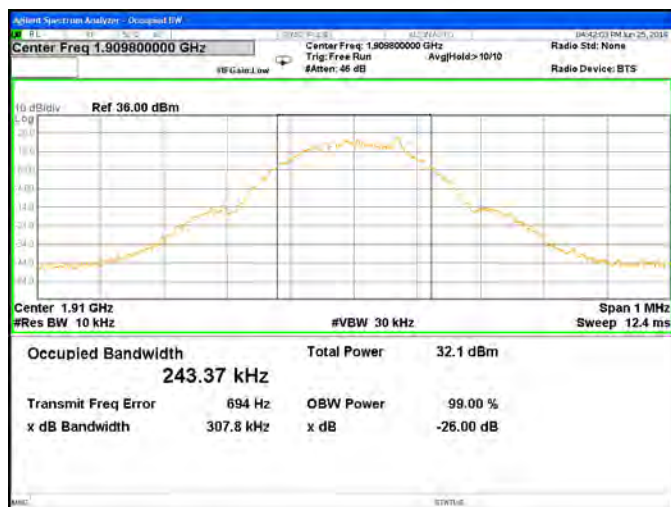
PCS 1900 CH 810
