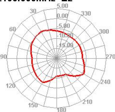
2100.000MHz E2
