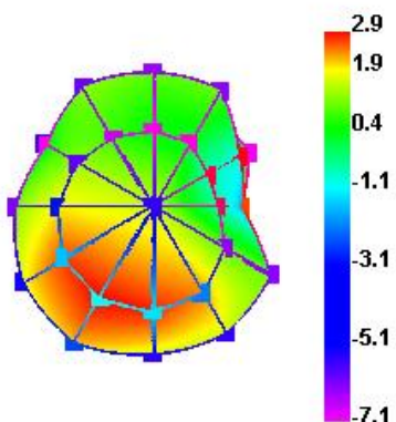
1575.000MHz
