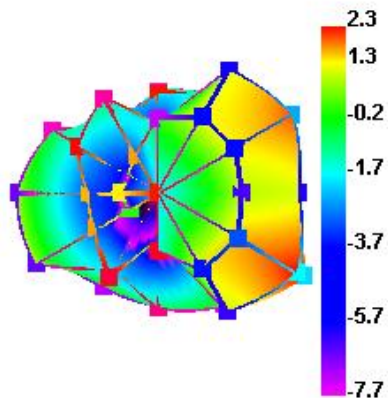
1575.000MHz
