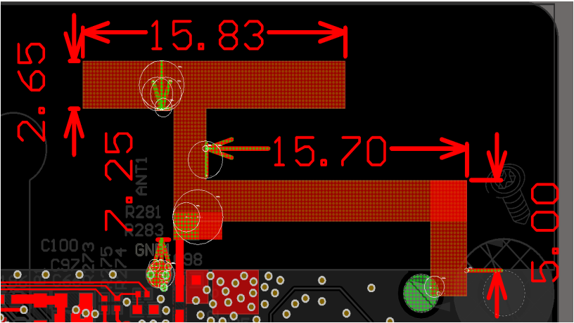
天线尺寸/ANT Size
