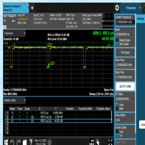
NTVN-11AC40SISO-Ant2-5755-0.65-0.69
