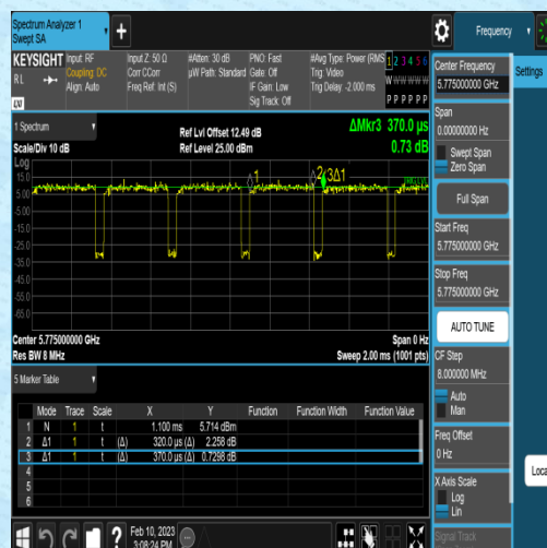
NTVN-11AC80SISO-Ant2-5775-0.32-0.37
