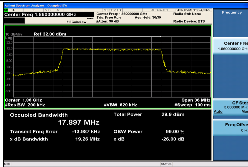
Band2-20MHz-QPSK-18700-100RB#0-17.897
