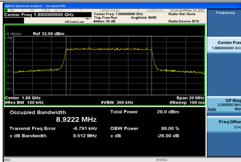
Band2-10MHz-QPSK-18900-50RB#0-8.9222
