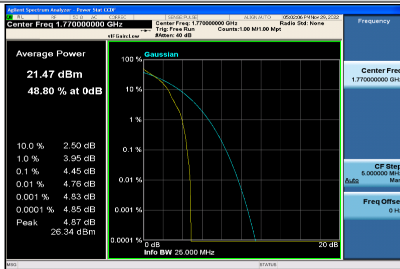
Band66-20MHz-QPSK-132572-1RB#0
