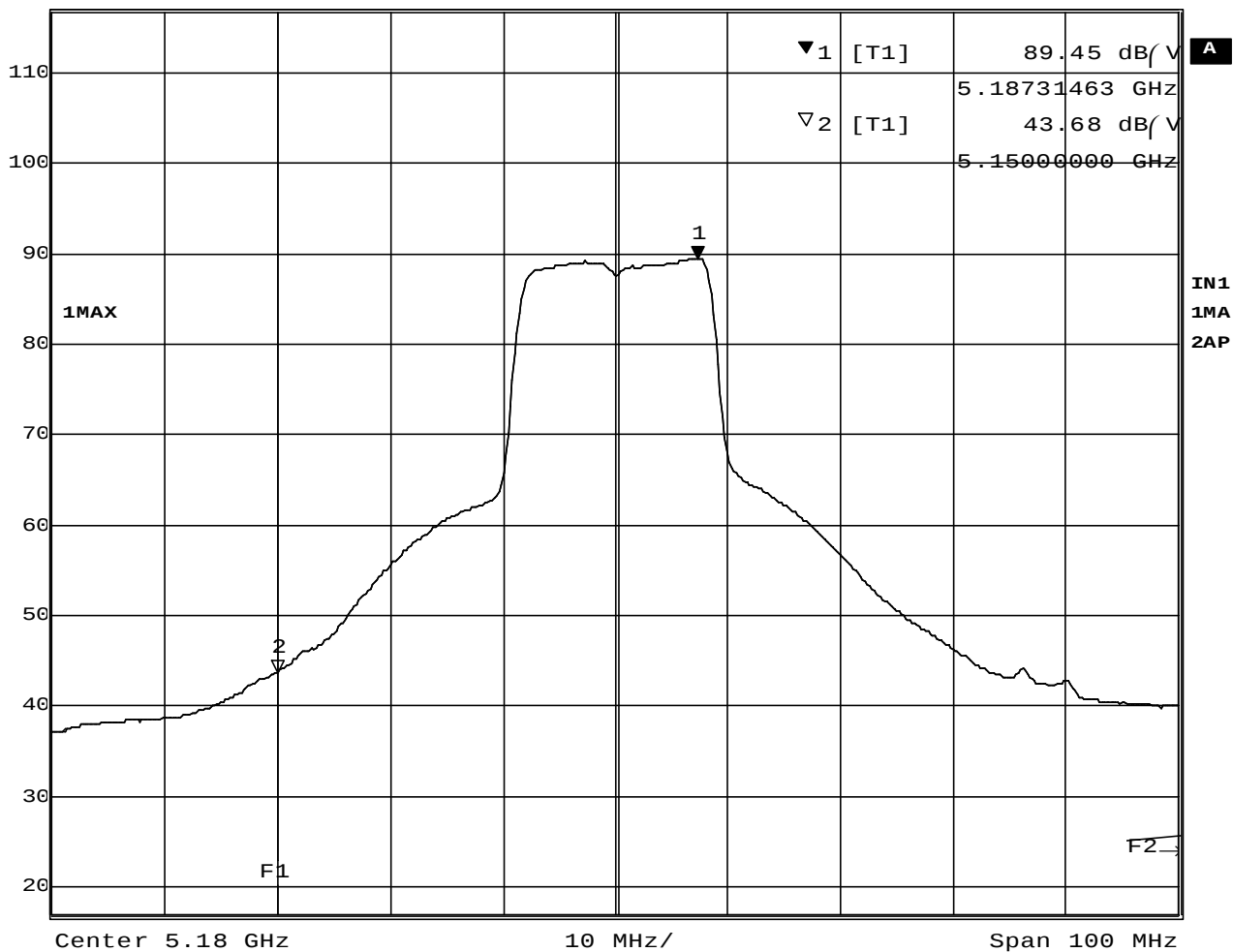
Plot 7-1-2 5180MHz TX mode (Average)
