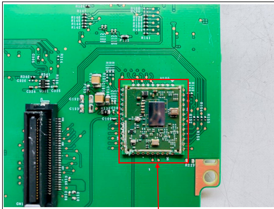
BT/WIFI Module
