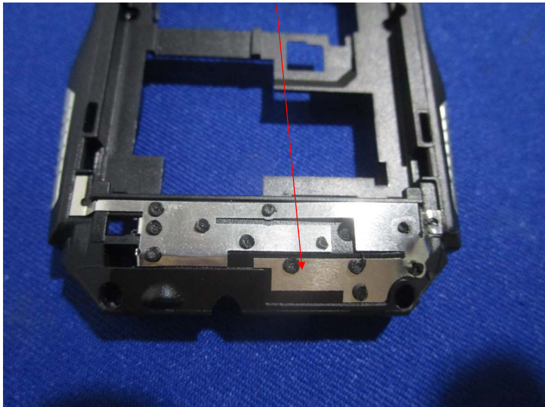
GSM ANT
