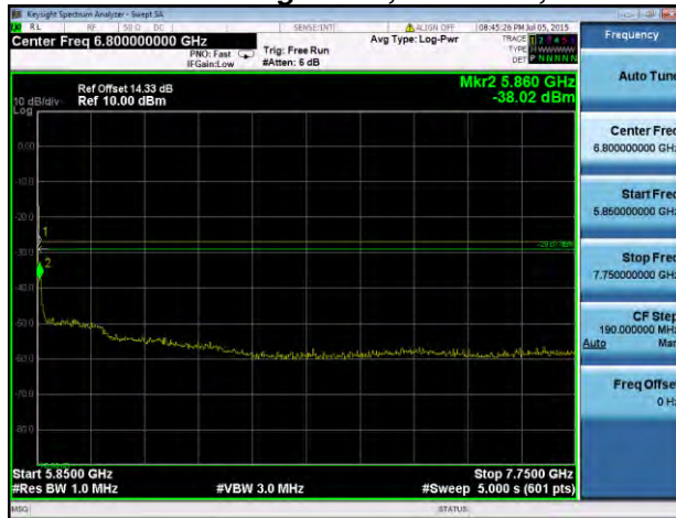
Antenna A
