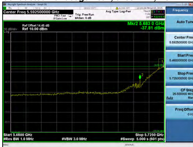
Antenna A
