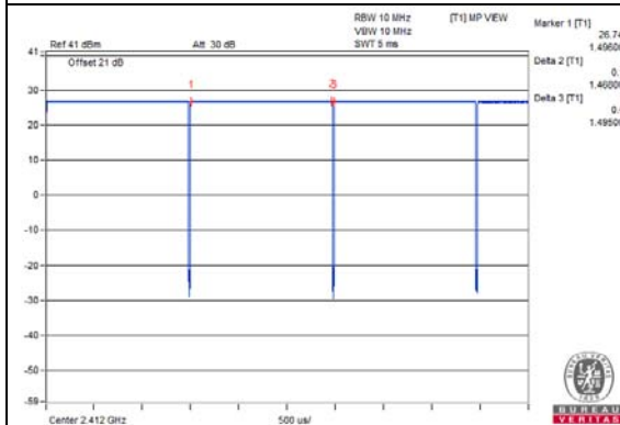
802.11ax (HE20)
