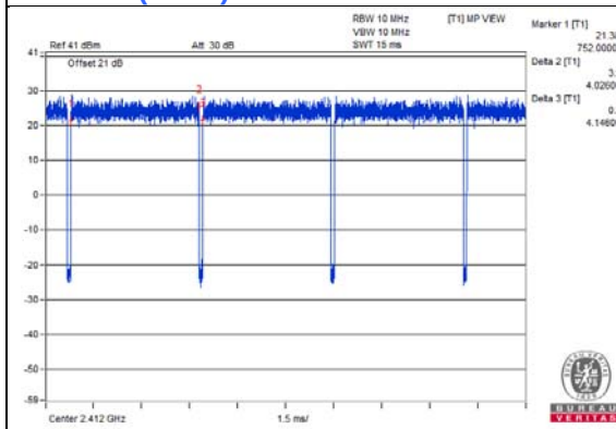
802.11ax (HE20)
