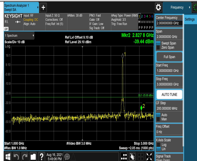
Band7-10MHz-QPSK-21400-50RB#0-Range2:1000~3000MHz
