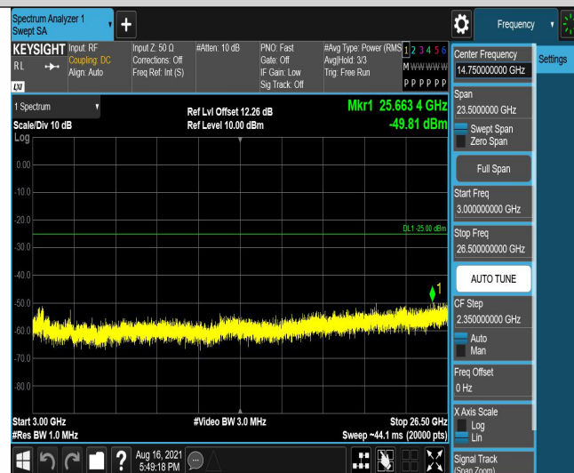
Band7-10MHz-QPSK-21400-50RB#0-Range3:3000~26500MHz
