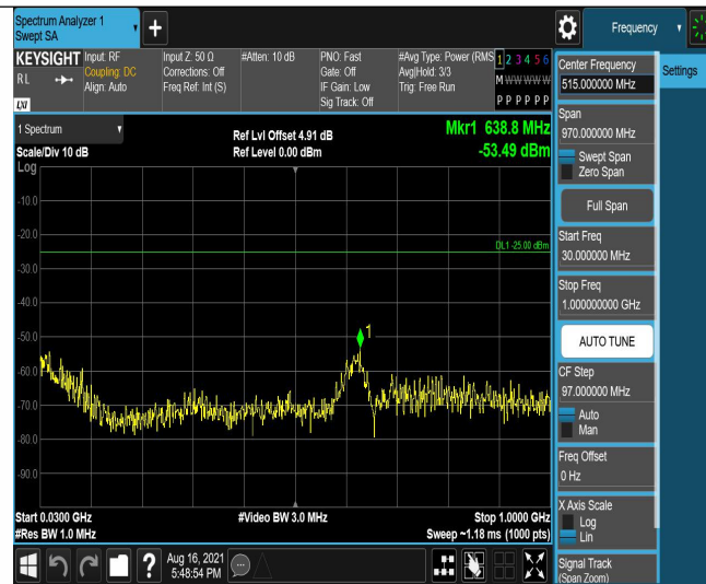
Band7-10MHz-QPSK-21400-50RB#0-Range1:30~1000MHz
