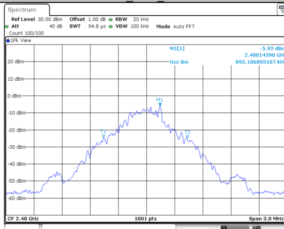
DH5_Ant1_2480
