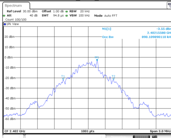
DH5_Ant1_2402
