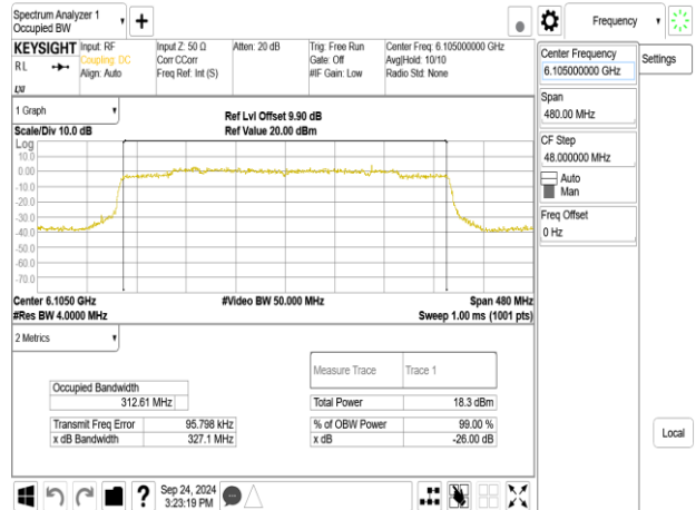
802.11be_320MHz_ChainA_6105MHz_2x996+484_MRUC2
