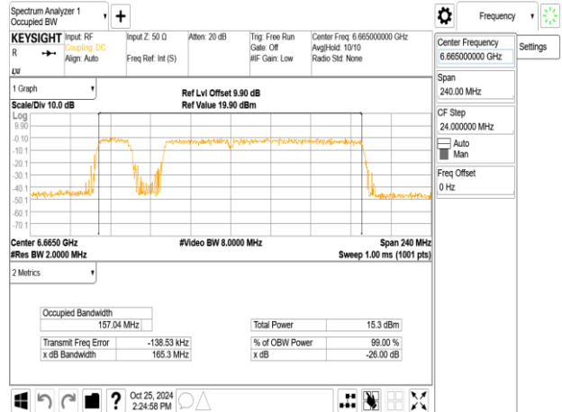
802.11be_160MHz_ChainB_6665MHz_996+484+242_MRU4
