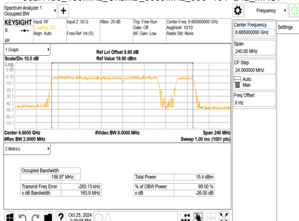
802.11be_160MHz_ChainB_6665MHz_996+484+242_MRU8
