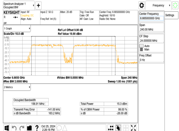
802.11be_160MHz_ChainB_6665MHz_996+484+242_MRU5
