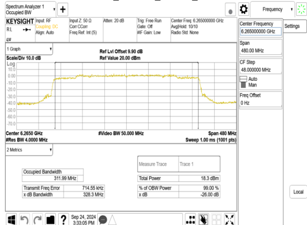
802.11be_320MHz_ChainA_6265MHz
