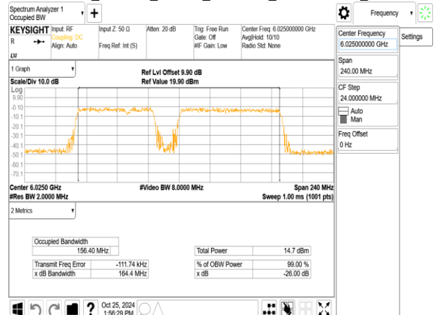
802.11be_160MHz_ChainB_6025MHz_996+484+242_MRU4
