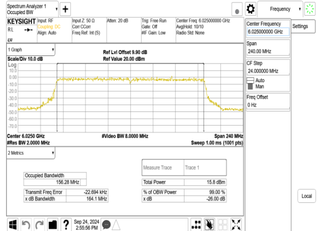
802.11be_160MHz_ChainB_6025MHz_996+484+242_MRU2
