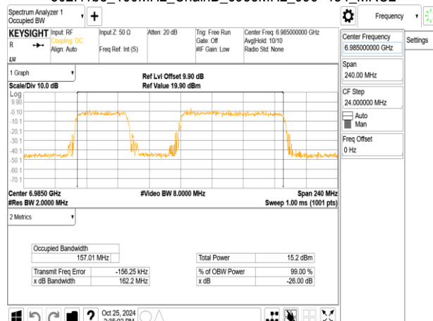
802.11be_160MHz_ChainB_6985MHz_996+484_MRU2
