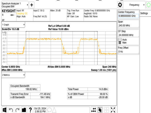
802.11be_160MHz_ChainB_6985MHz_996+484_MRUC4
