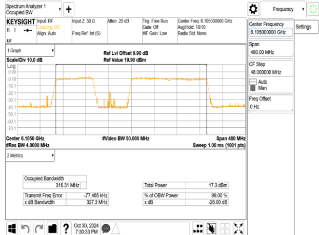
802.11be_320MHz_ChainA_6105MHz_3x996_MRUE
