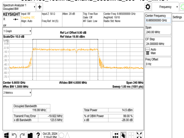
802.11be_160MHz_ChainB_6665MHz_996+484_MRU4
