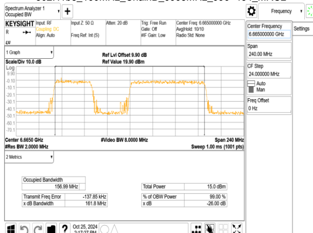
802.11be_160MHz_ChainB_6665MHz_996+484_MRU3
