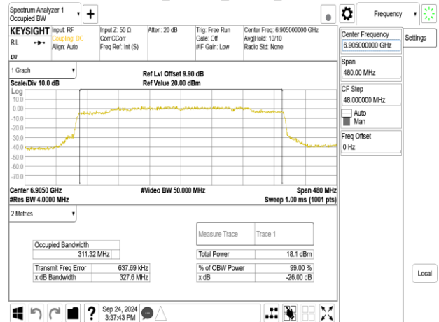
802.11be_320MHz_ChainA_6905MHz_3x996+484_MRU1
