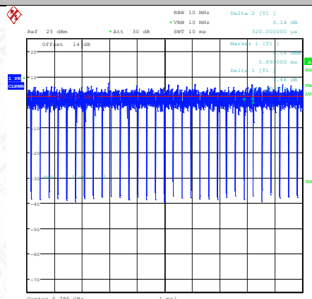
NTNV-11AX40MIMO-Ant2-5795
