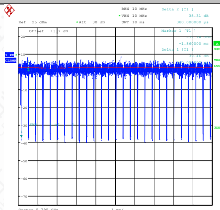
NTNV-11AC40MIMO-Ant1-5795
