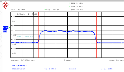
11AX40MIMO-Ant1-5755-PASS
