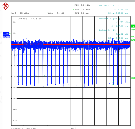
NTNV-11AC80SISO-Ant1-5775
