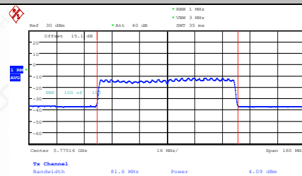
11AX80SISO-Ant2-5775-PASS
