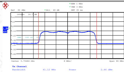
11AX40MIMO-Ant1-5795-PASS
