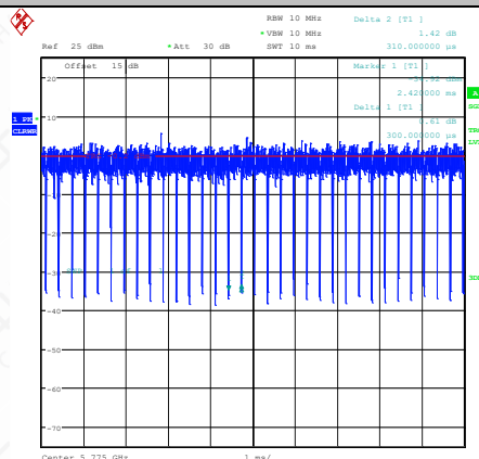
NTNV-11AX80SISO-Ant2-5775
