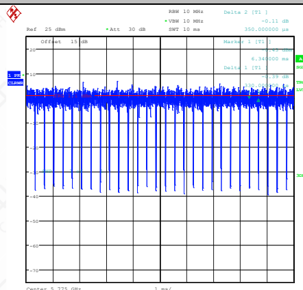
NTNV-11AC80SISO-Ant2-5775
