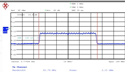
11AX80SISO-Ant1-5775-PASS
