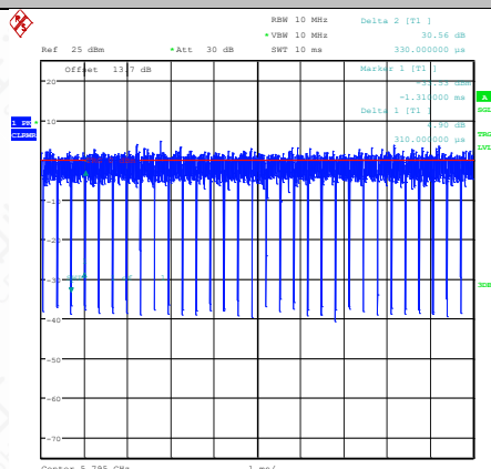
NTNV-11AX40MIMO-Ant1-5795
