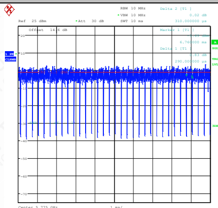
NTNV-11AX80SISO-Ant1-5775
