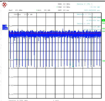
NTNV-11AX40MIMO-Ant1-5755
