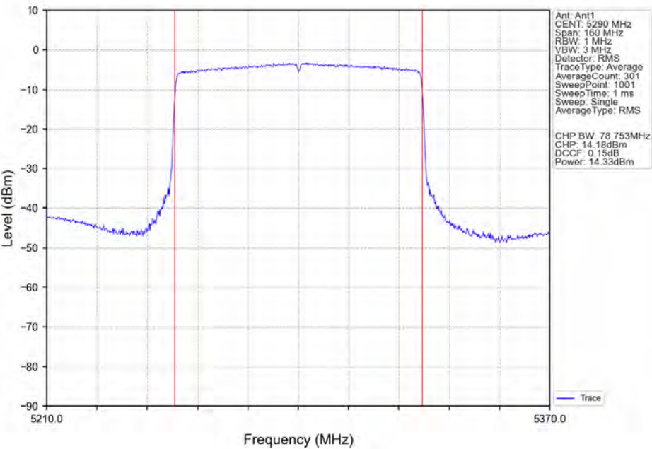
802.11ax(HE80)_MCH_5290MHz_RU996_Left_Ant1_NTNV
