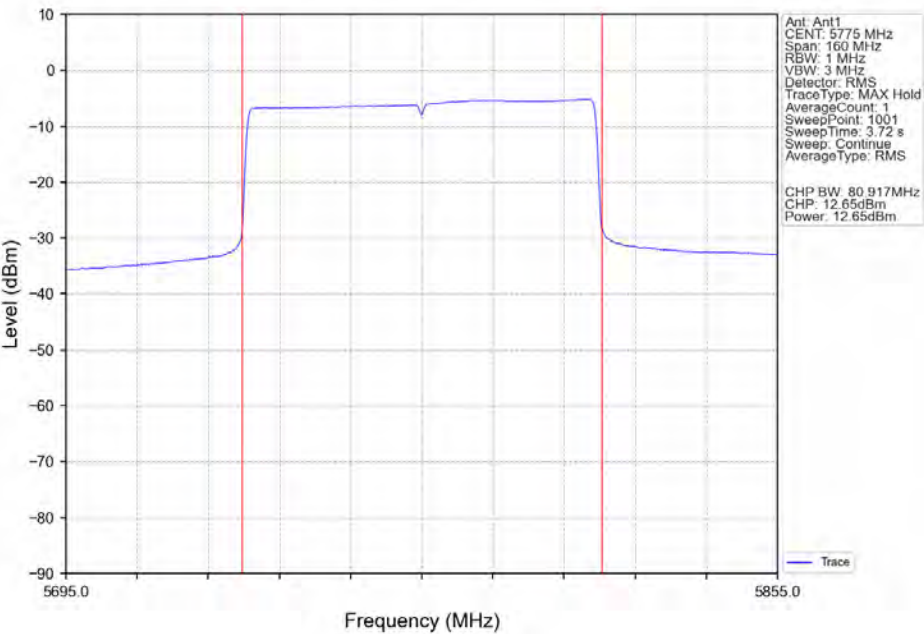
802.11ax(HE80)_MCH_5775MHz_RU996_Left_Ant1_NTNV
