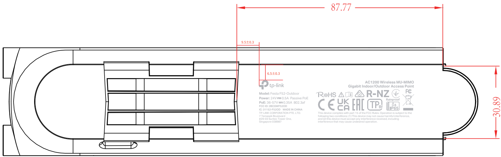
尺寸图
