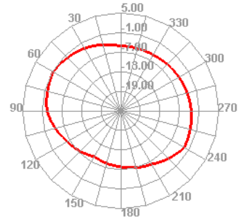
2480.000MHz H
