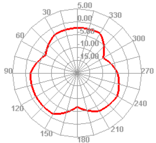
2440.000MHz E2
