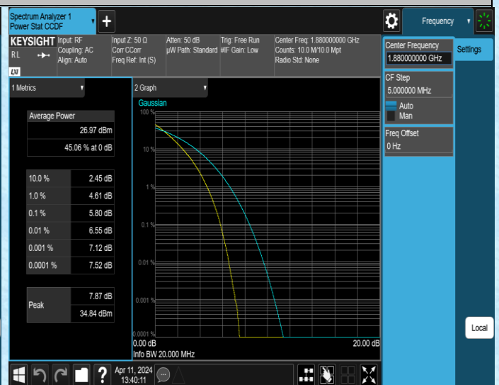
Band2-20MHz-QPSK-18900-100RB#0-PASS
