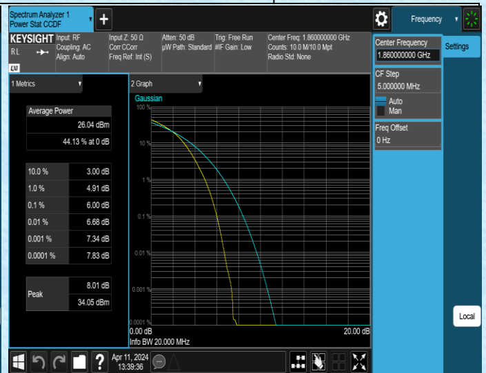
Band2-20MHz-16QAM-18700-100RB#0-PASS
