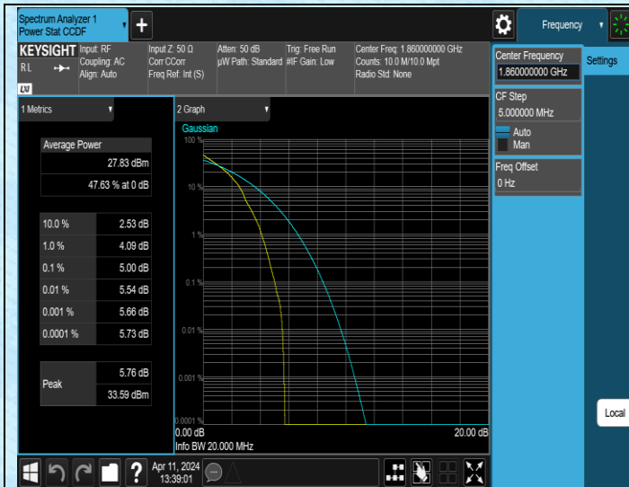
Band2-20MHz-QPSK-18700-1RB#0-PASS
