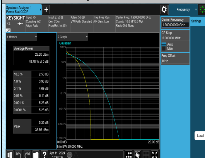
Band2-20MHz-QPSK-19100-1RB#0-PASS
