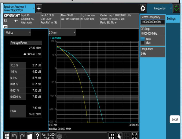
Band2-20MHz-QPSK-19100-100RB#0-PASS
