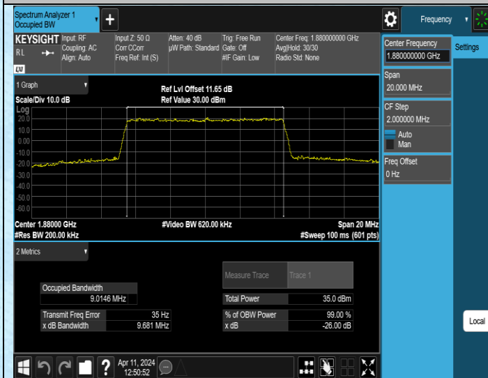
Band2-10MHz-16QAM-18900-50RB#0-PASS
