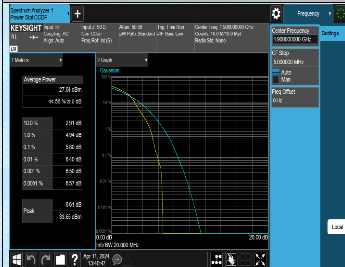
Band2-20MHz-16QAM-19100-1RB#0-PASS
