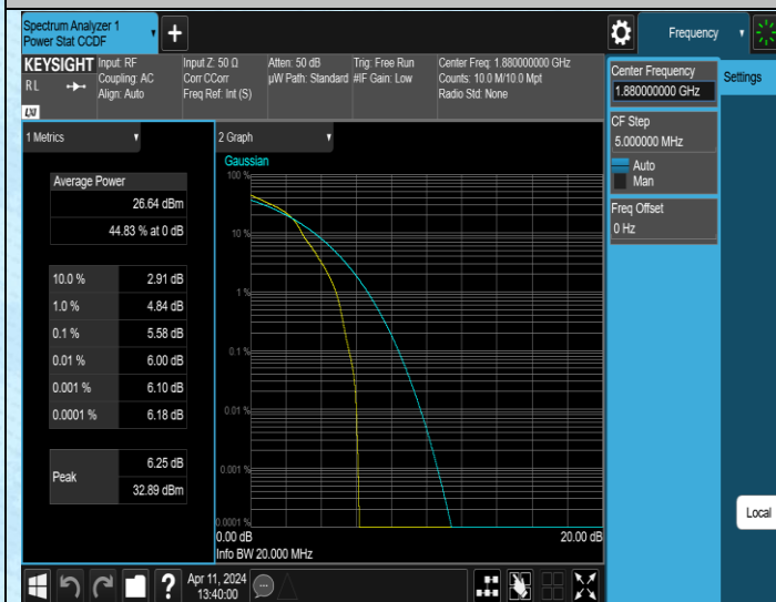
Band2-20MHz-16QAM-18900-1RB#0-PASS
