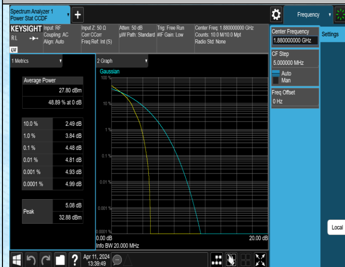
Band2-20MHz-QPSK-18900-1RB#0-PASS
