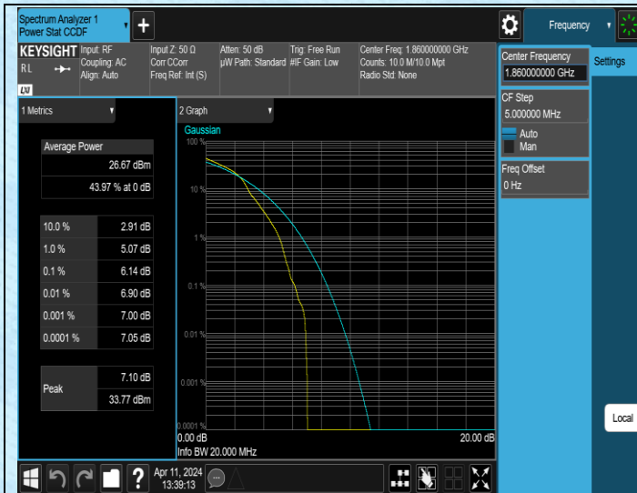
Band2-20MHz-16QAM-18700-1RB#0-PASS
