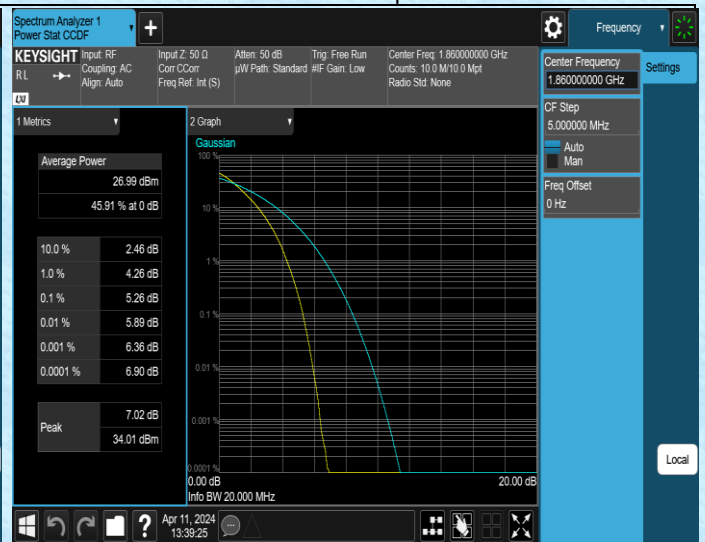
Band2-20MHz-QPSK-18700-100RB#0-PASS
