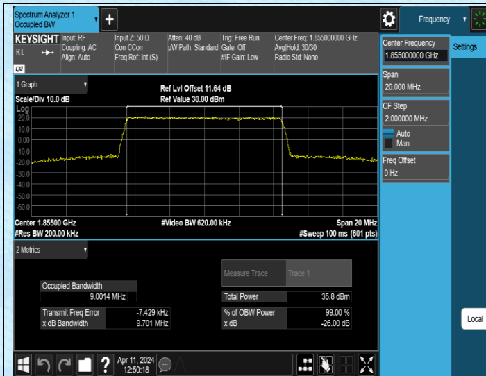
Band2-10MHz-QPSK-18650-50RB#0-PASS
