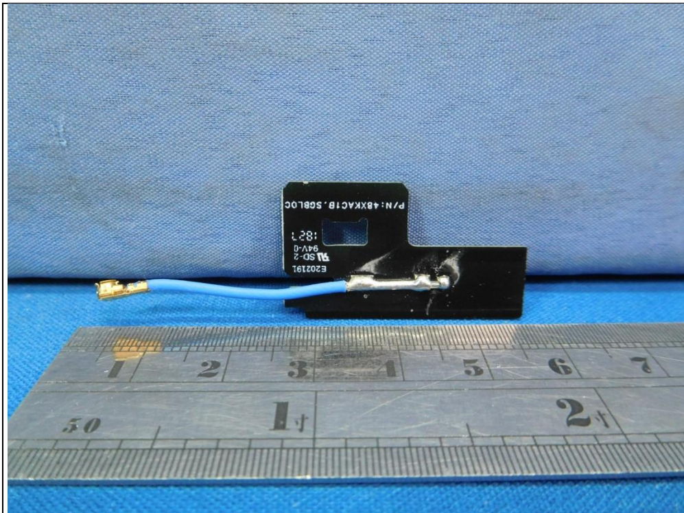
Antenna: 5GH1
