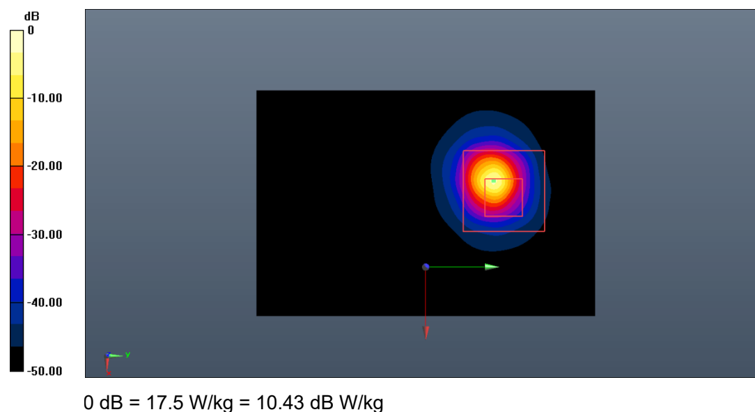
Fig.B.12. Validation 5250MHz 100mW
