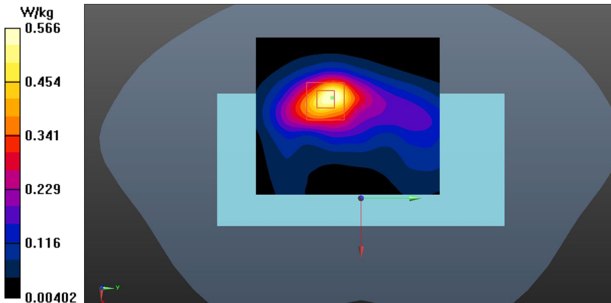
Fig.34 NR n38 Body
