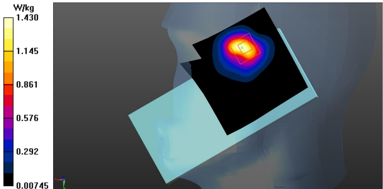
Fig.33 NR n38 Head
