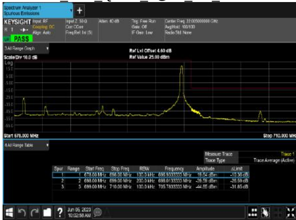
B71 20M 16QAM 1@99 CH 133372
