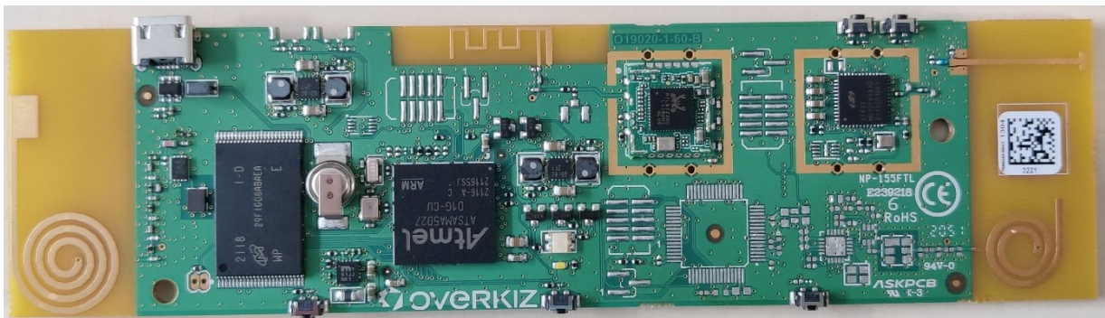
EUT PCB Top Side
