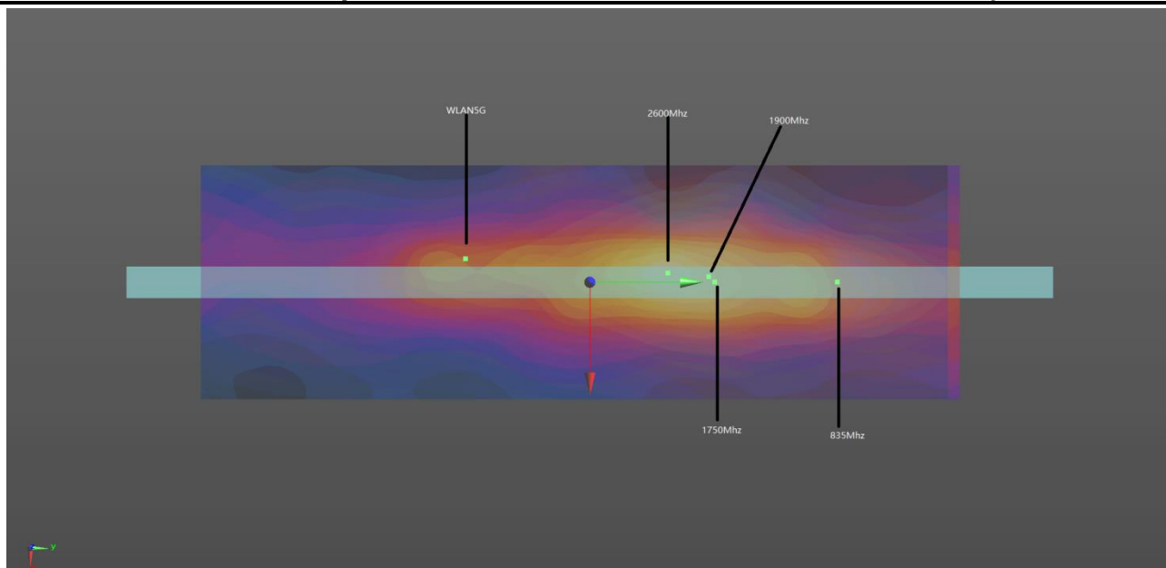
WWAN+WLAN 5GHz Edge 1
