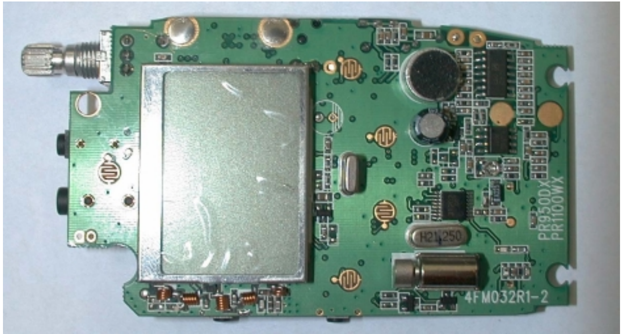
PCB Top
