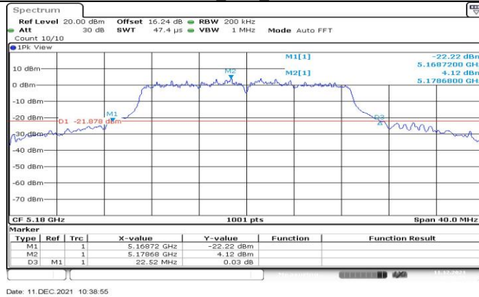
11AC20MIMO_Ant1_5180
