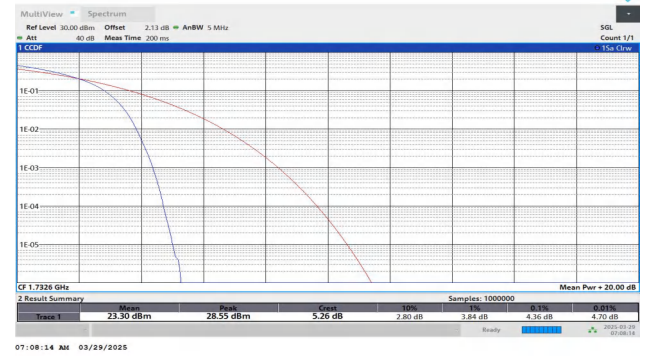
Band4-1413-5-PASS
