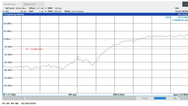
Band4-1312-1-PASS
