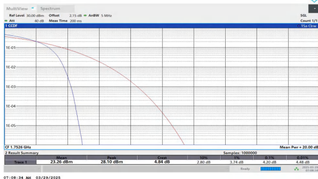
Band4-1513-5-PASS
