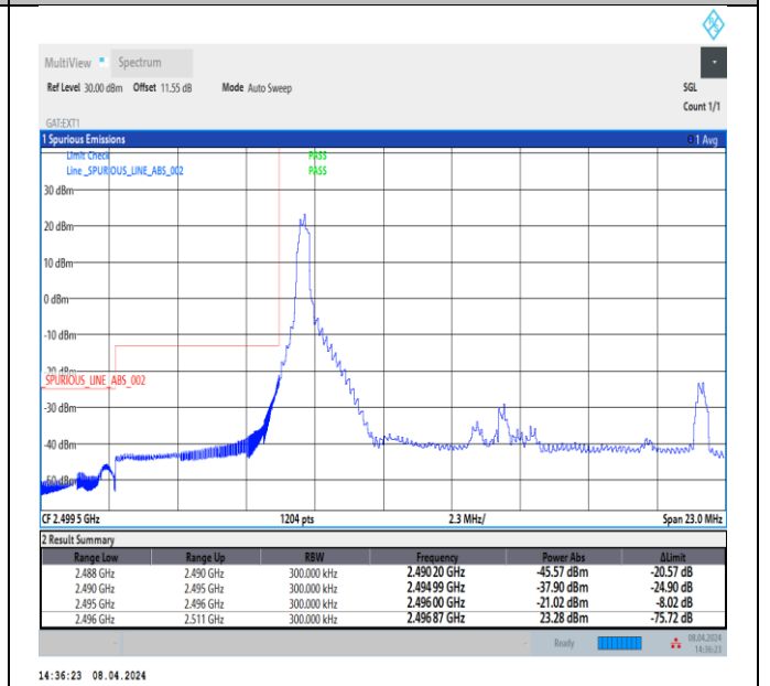
Band41_15MHz_QPSK_39725_1RB#0
