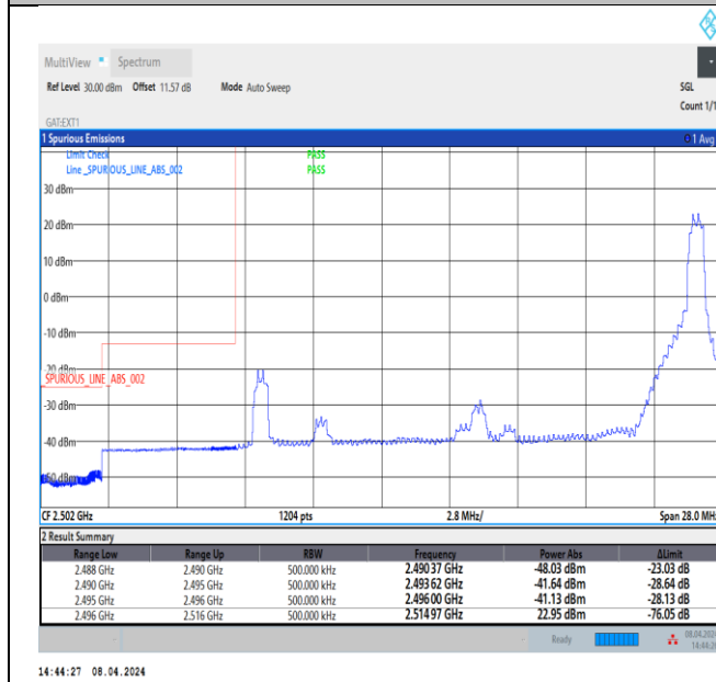
Band41_20MHz_QPSK_39750_1RB#99
