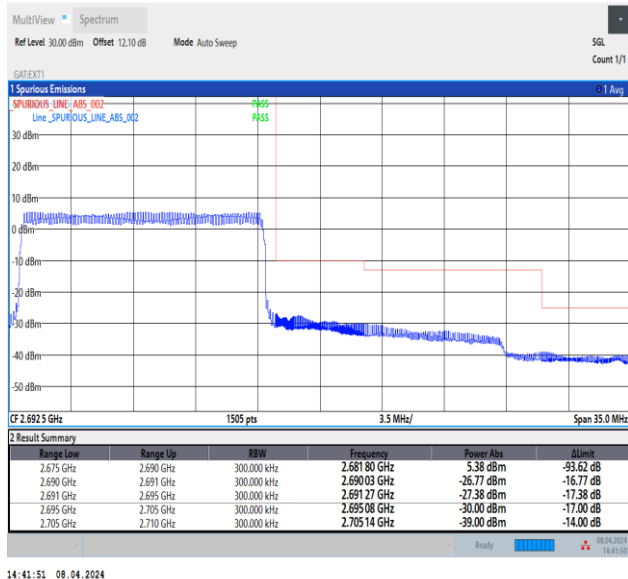
Band41_15MHz_QPSK_41515_75RB#0
