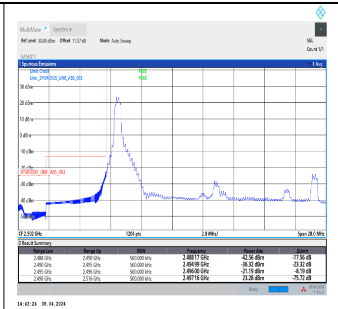
Band41_20MHz_QPSK_39750_1RB#0
