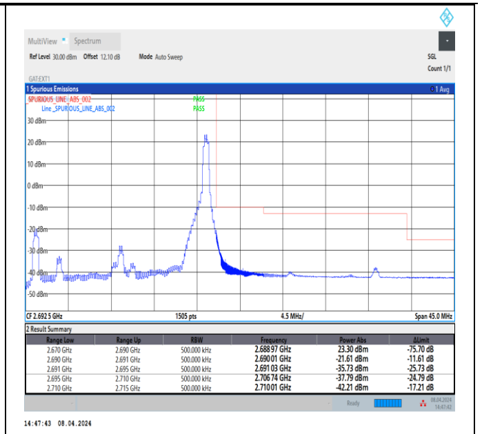
Band41_20MHz_QPSK_41490_1RB#99
