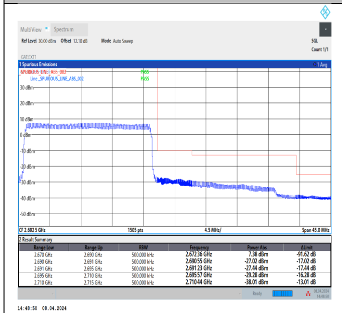
Band41_20MHz_QPSK_41490_100RB#0
