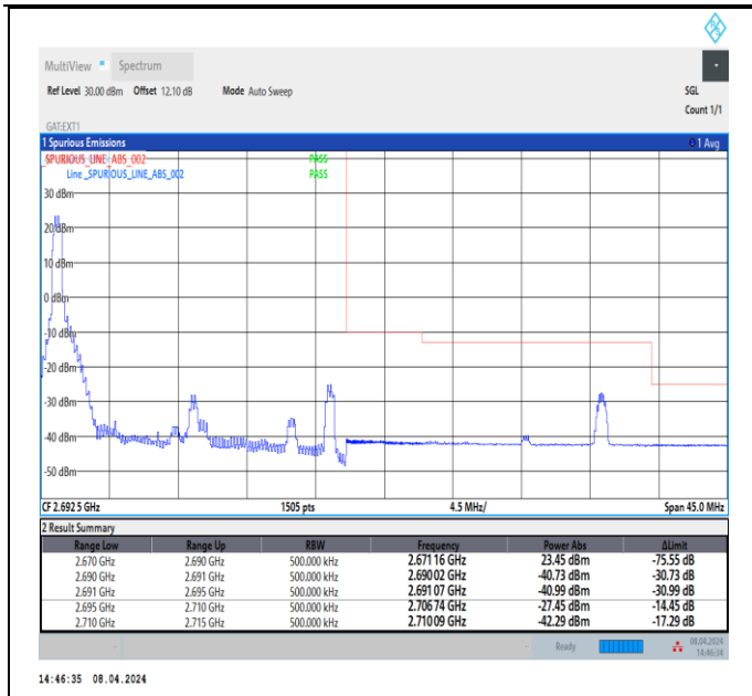
Band41_20MHz_QPSK_41490_1RB#0
