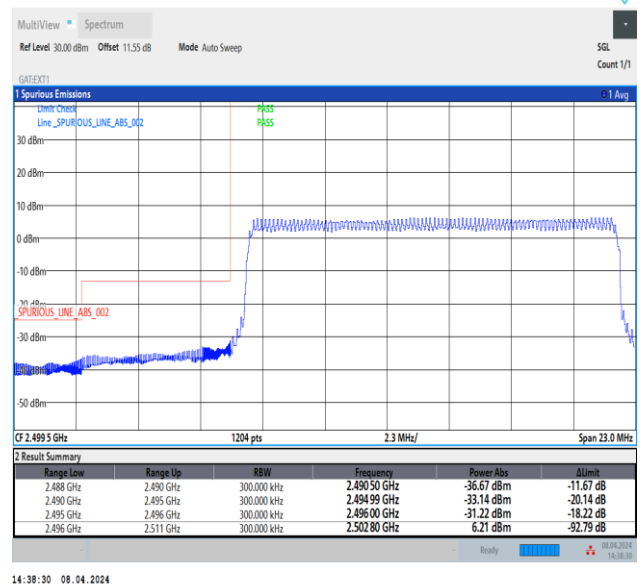
Band41_15MHz_QPSK_39725_75RB#0
