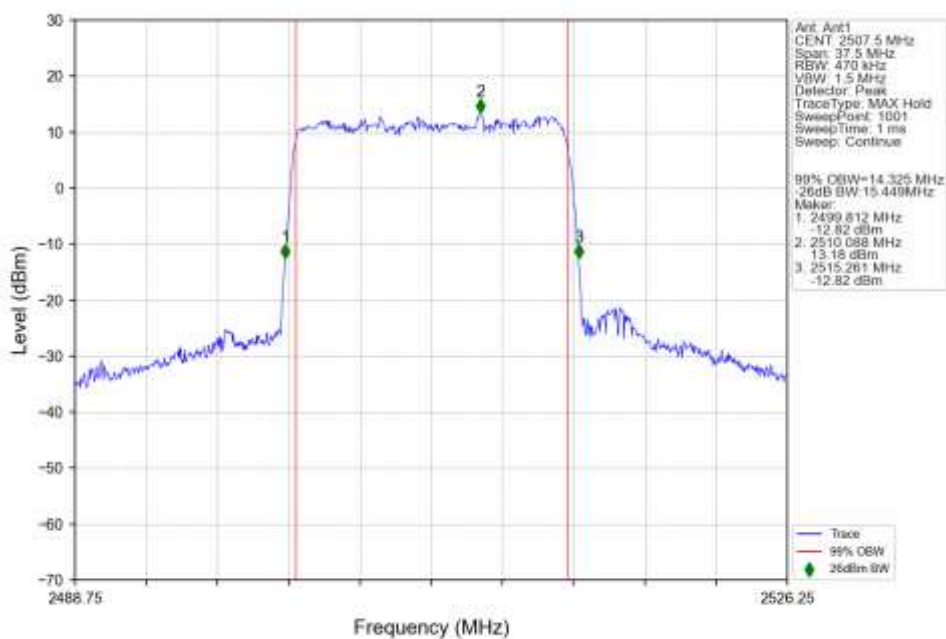
n7_15kHz_SISO_NTNV_15MHz_CP-OFDM_256_QAM_2507.5MHz_Outer_Full_Ant1
