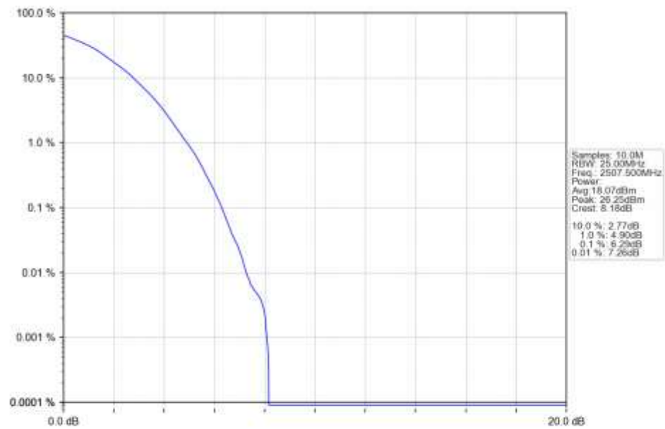
n7_15kHz_SISO_NTNV_15MHz_DFT-s-OFDM_256_QAM_2507.5MHz_Outer_Full_Ant1
