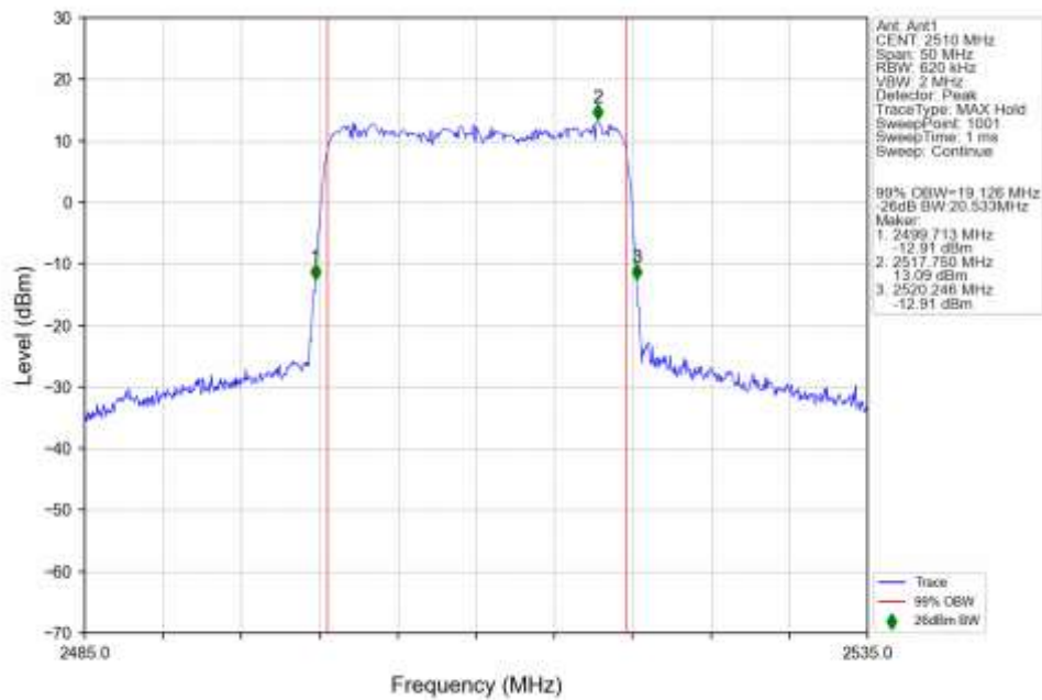
n7_15kHz_SISO_NTNV_20MHz_CP-OFDM_256_QAM_2510MHz_Outer_Full_Ant1
