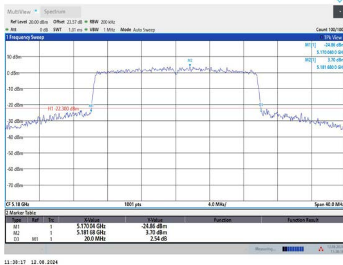
11BE20MIMO_Ant2_5180
