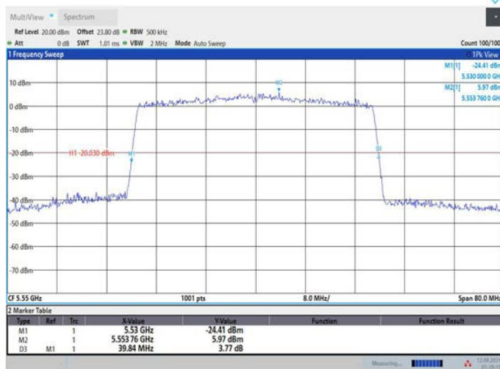
11AX40MIMO_Ant3_5550
