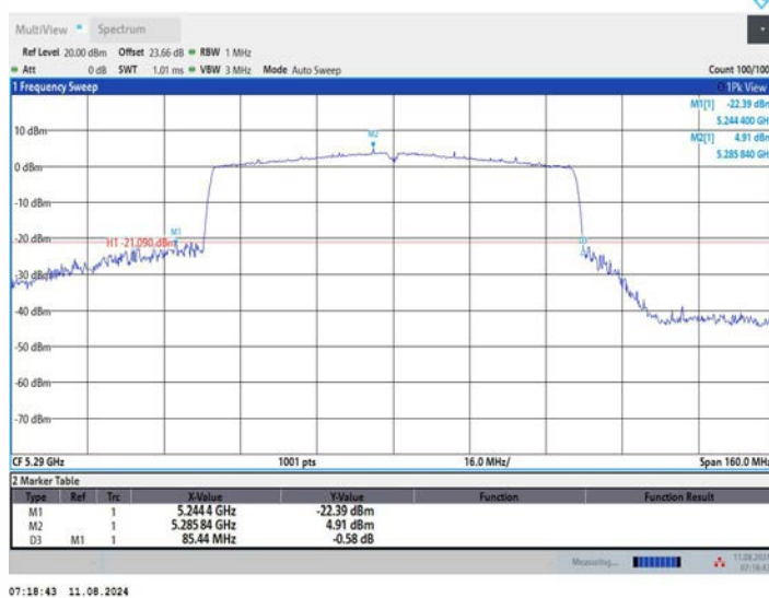
11AC80MIMO_Ant2_5290
