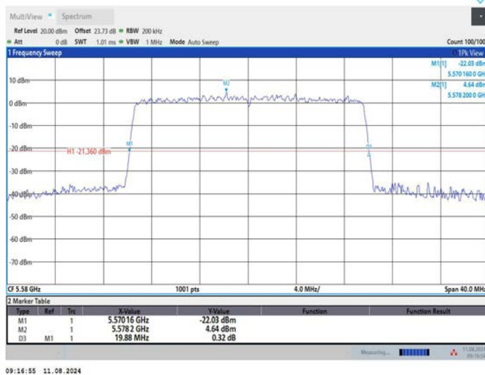
11AX20MIMO_Ant3_5580
