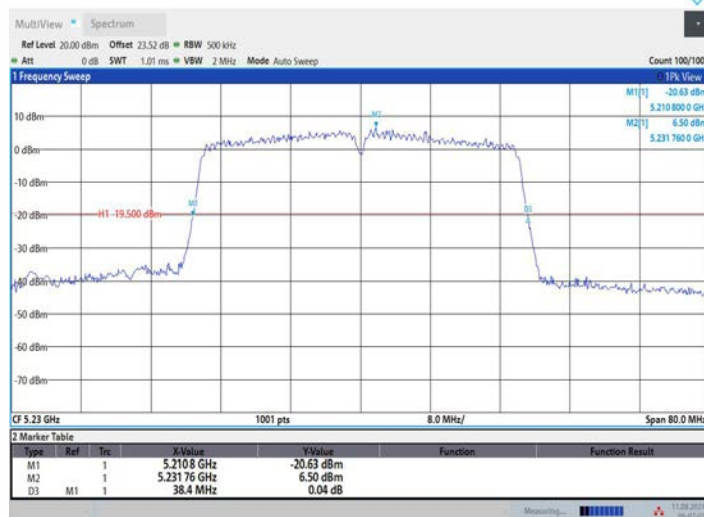
11AC40MIMO_Ant3_5230
