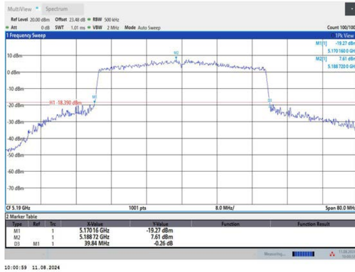
11AX40MIMO_Ant3_5190
