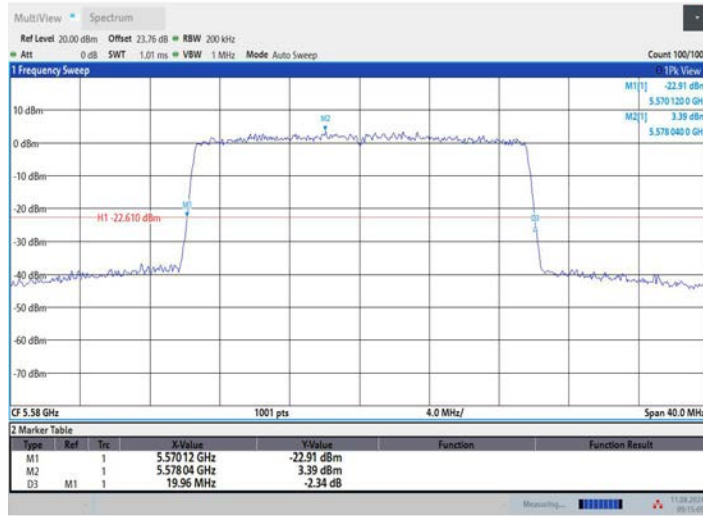
11AX20MIMO_Ant2_5580
