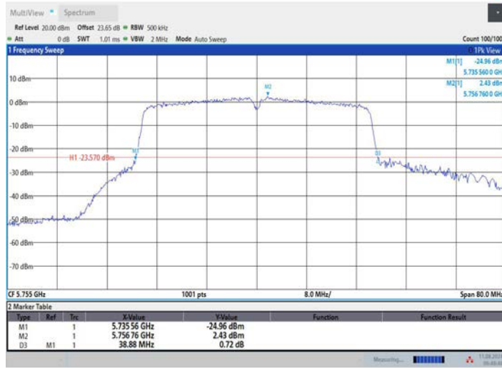
11AC40MIMO_Ant2_5755
