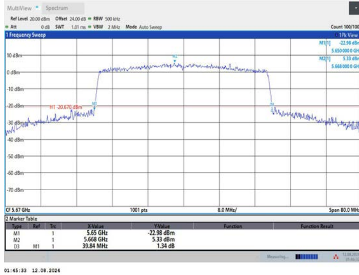
11AX40MIMO_Ant3_5670
