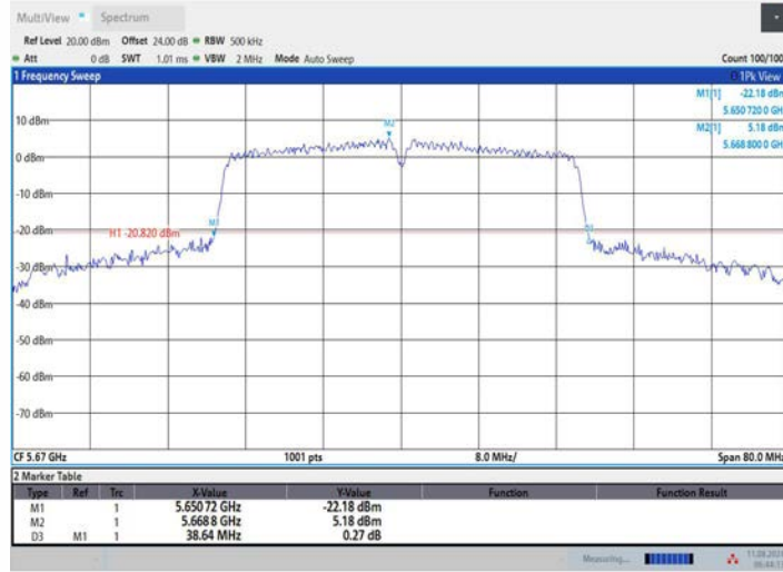
11AC40MIMO_Ant3_5670
