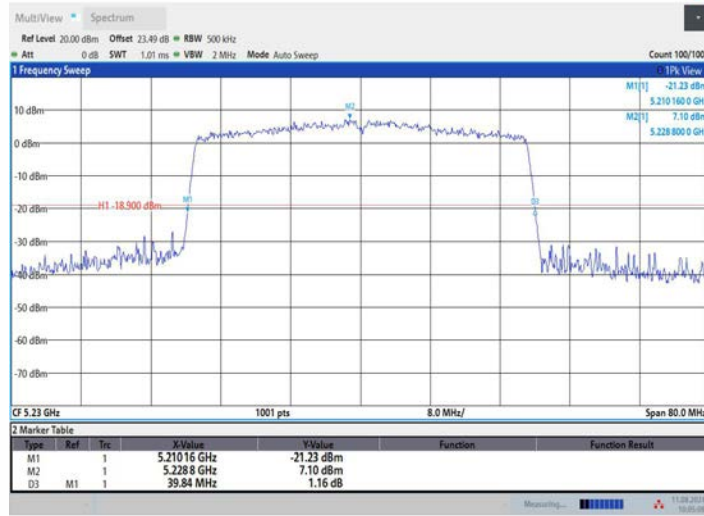
11AX40MIMO_Ant2_5230
