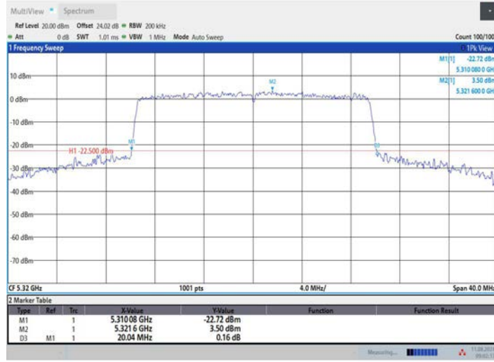
11AX20MIMO_Ant2_5320
