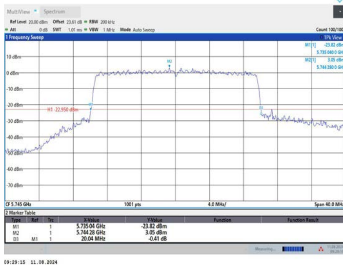
11AX20MIMO_Ant3_5745
