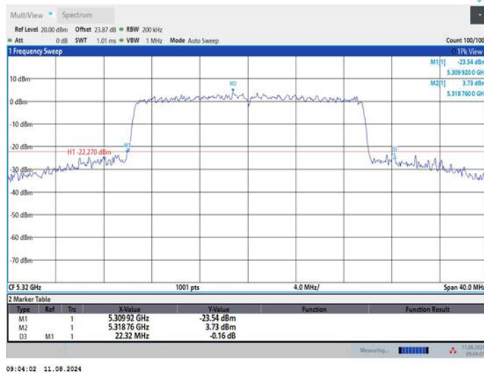
11AX20MIMO_Ant3_5320
