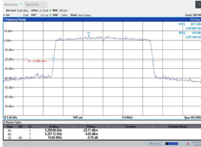
11BE20MIMO_Ant2_5260
