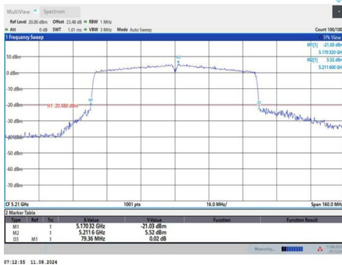
11AC80MIMO_Ant3_5210
