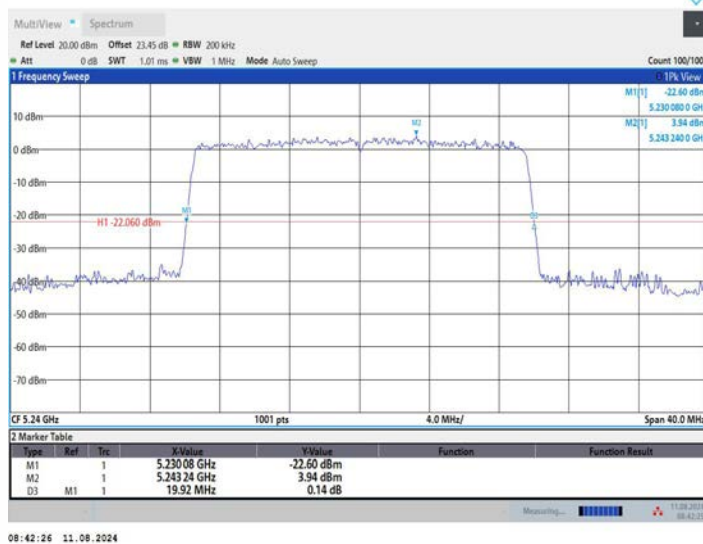
11AX20MIMO_Ant2_5240
