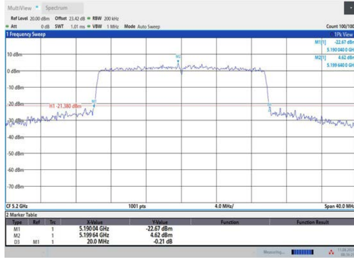
11AX20MIMO_Ant2_5200
