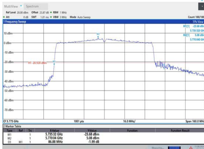
11AC80MIMO_Ant3_5775
