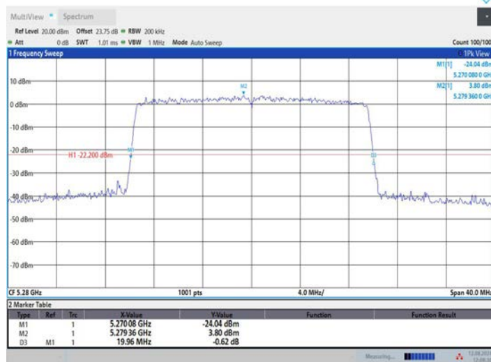
11BE20MIMO_Ant2_5280
