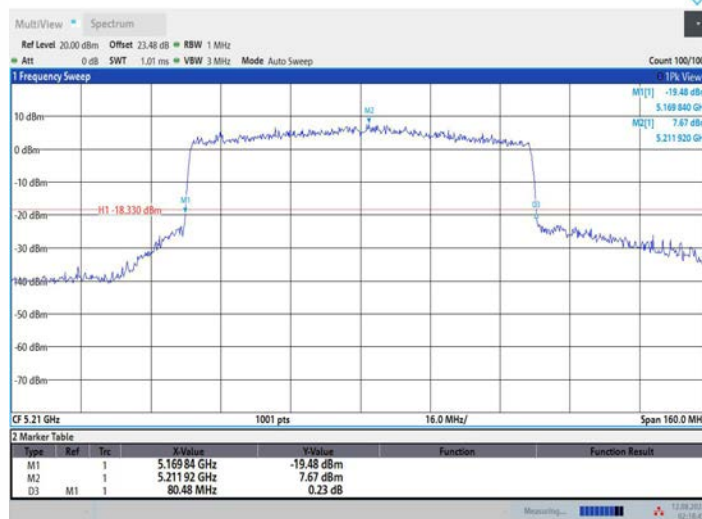
11AX80MIMO_Ant3_5210
