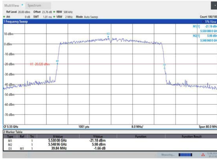
11AX40MIMO_Ant2_5550
