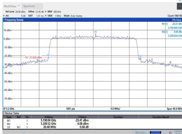
11AX20MIMO_Ant3_5200
