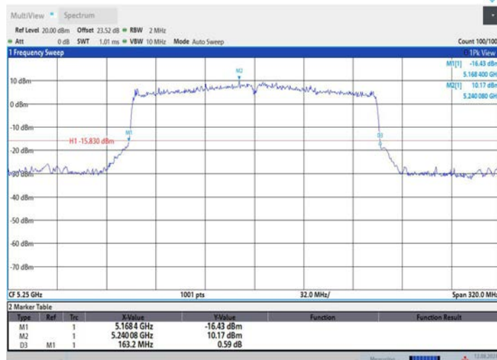
11AX160MIMO_Ant2_5250
