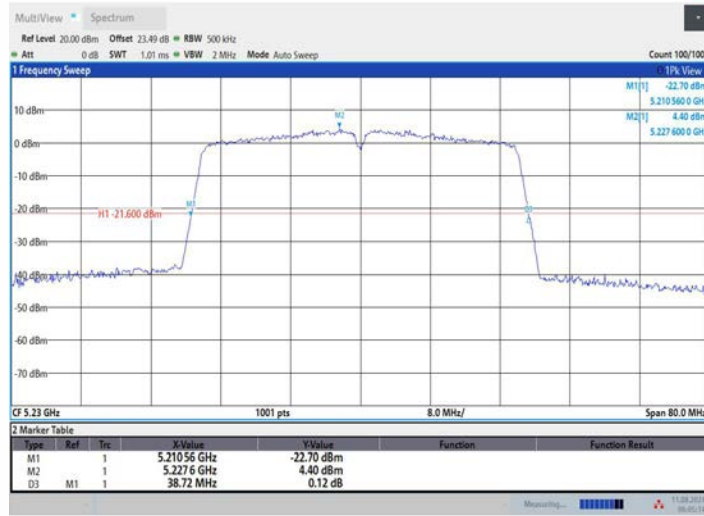
11AC40MIMO_Ant2_5230
