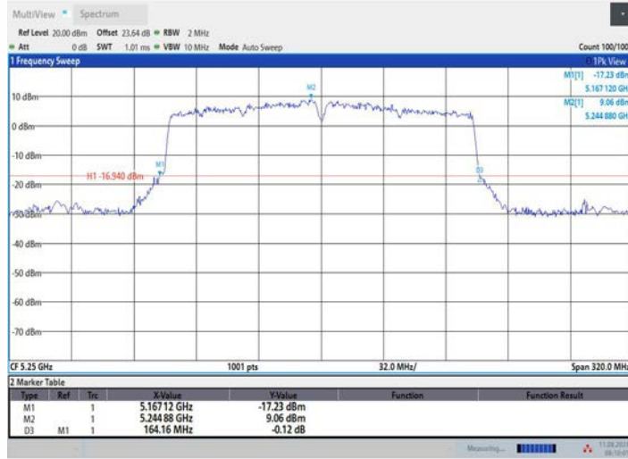
11AC160MIMO_Ant3_5250
