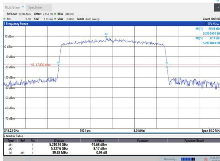
11AX40MIMO_Ant3_5230
