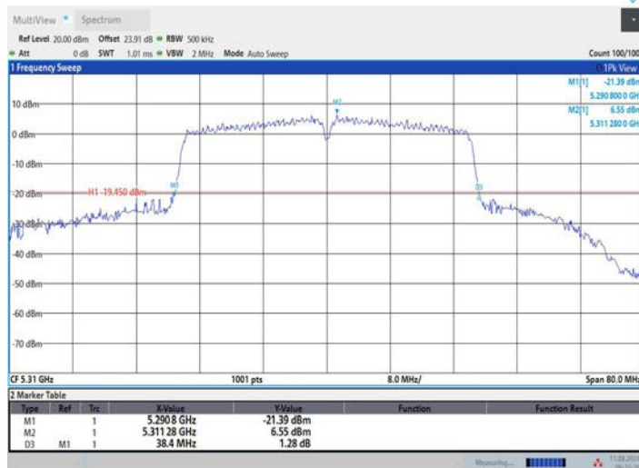
11AC40MIMO_Ant3_5310
