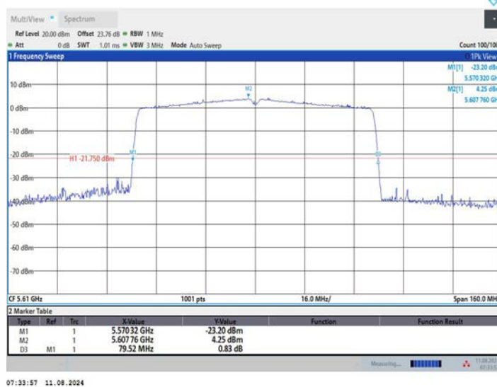
11AC80MIMO_Ant2_5610
