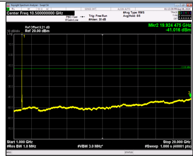
2-2-20MHz-20MHz-QPSK-QPSK-18700-18898-1RB#99-0 RB#0-1000~20000MHz-PASS
