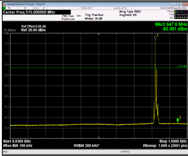
5-5-3MHz-5MHz-QPSK-QPSK-20416-20455-1RB#0-1R B#24-30~1000MHz-PASS
