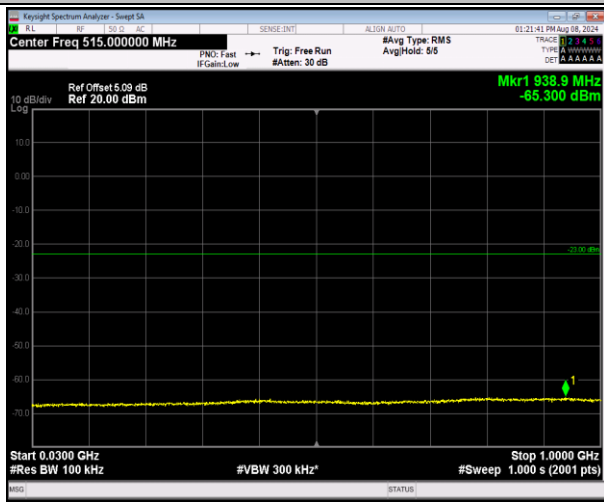
2-2-20MHz-20MHz-16QAM-16QAM-18801-18999-100RB#0-100RB#0-30~1000MHz-PASS
