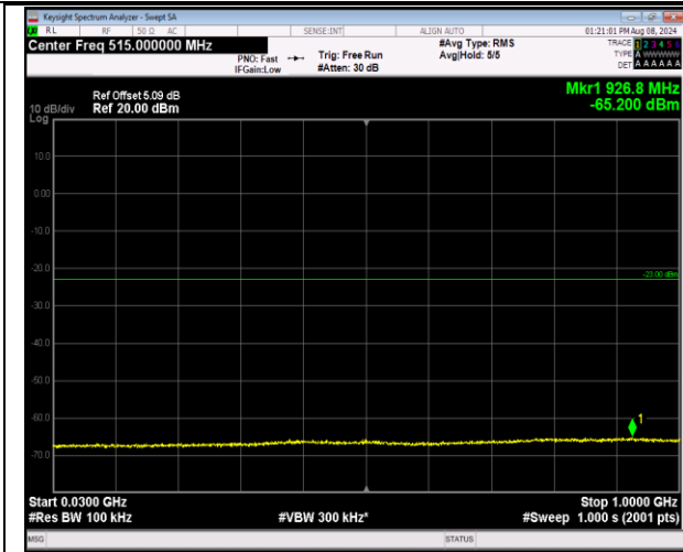
2-2-20MHz-20MHz-QPSK-QPSK-18801-18999-100RB# 0-100RB#0-30~1000MHz-PASS
