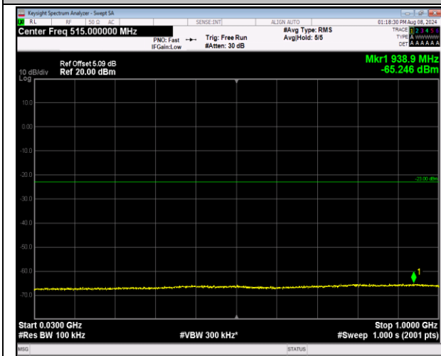
2-2-20MHz-20MHz-QPSK-QPSK-18801-18999-1RB#99-0 ORB#0-30~1000MHz-PASS
