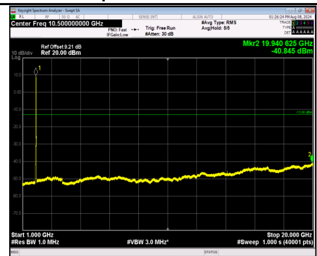
2-2-20MHz-20MHz-QPSK-QPSK-18902-19100-100RB#0- 100RB#0-1000~20000MHz-PASS
