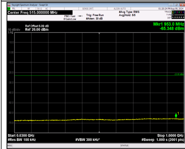
2-2-20MHz-20MHz-16QAM-16QAM-18801-18999-1RB# 0-1RB#99-30~1000MHz-PASS
