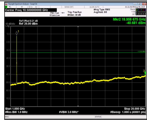
2-2-20MHz-20MHz-16QAM-16QAM-18801-18999-100RB#0-100RB#0-1000~20000MHz-PASS
