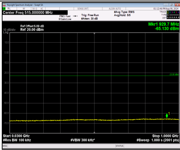
2-2-20MHz-20MHz-16QAM-16QAM-18700-18898-1RB# 0-0RB#0-30~1000MHz-PASS
