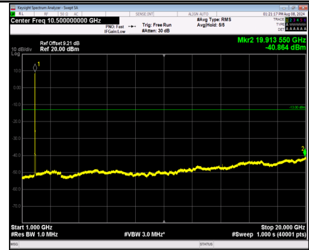
2-2-20MHz-20MHz-QPSK-QPSK-18801-18999-100RB#0- 100RB#0-1000~20000MHz-PASS
