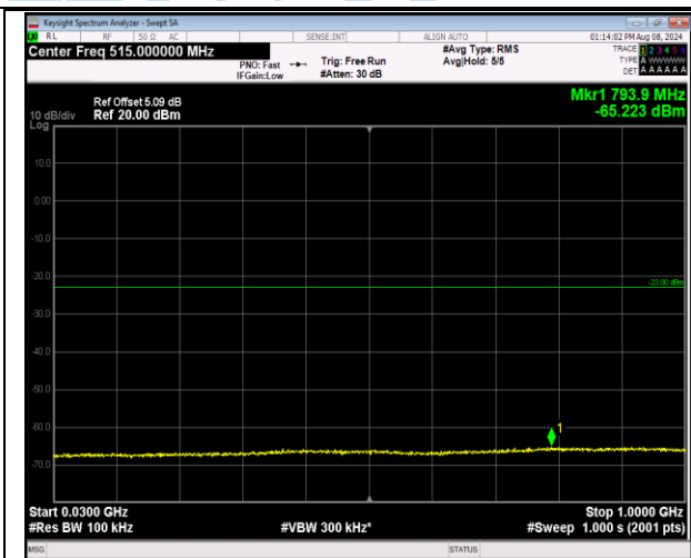
2-2-20MHz-20MHz-16QAM-16QAM-18700-18898-1RB# 99-0RB#0-30~1000MHz-PASS
