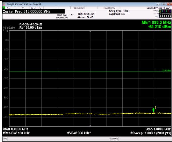
2-2-20MHz-20MHz-16QAM-16QAM-18700-18898-1RB# 0-1RB#99-30~1000MHz-PASS
