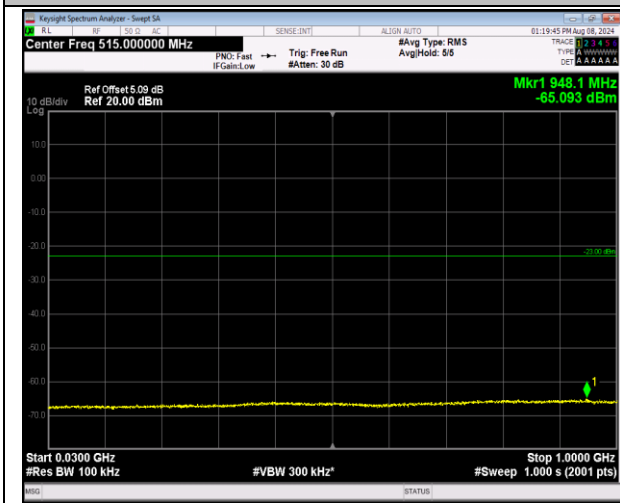
2-2-20MHz-20MHz-QPSK-QPSK-18801-18999-1RB#0-1 RB#99-30~1000MHz-PASS
