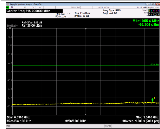
2-2-20MHz-20MHz-QPSK-QPSK-18700-18898-1RB#99-0 ORB#0-30~1000MHz-PASS
