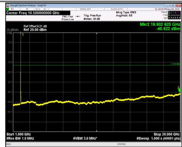
2-2-20MHz-20MHz-QPSK-QPSK-18801-18999-1RB#99-0 RB#0-1000~20000MHz-PASS
