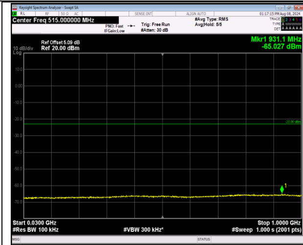
2-2-20MHz-20MHz-QPSK-QPSK-18801-18999-1RB#0-0 RB#0-30~1000MHz-PASS
