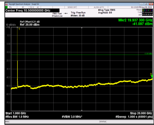
2-2-20MHz-20MHz-16QAM-16QAM-18700-18898-1RB#0 -0RB#0-1000~20000MHz-PASS
