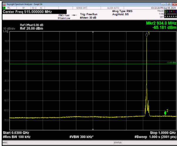
5-5-3MHz-5MHz-QPSK-QPSK-20416-20455-1RB#14-0R B#0-30~1000MHz-PASS
