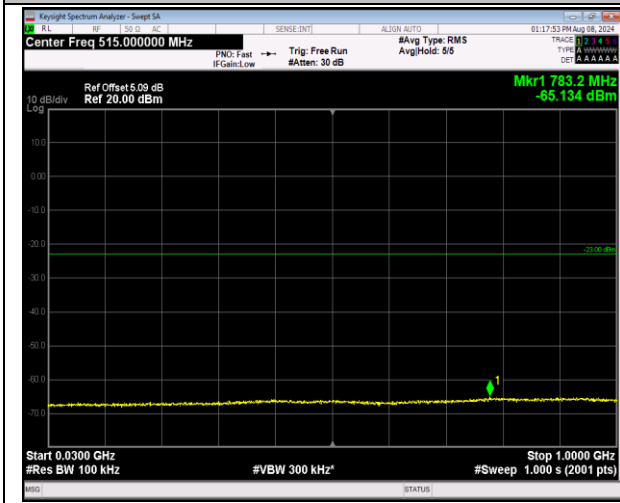
2-2-20MHz-20MHz-16QAM-16QAM-18801-18999-1RB# 0-0RB#0-30~1000MHz-PASS
