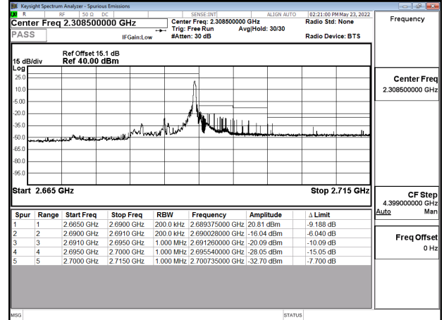
Emission Mask_Band41_10MHz_QPSK_RB1_49_CH41540
