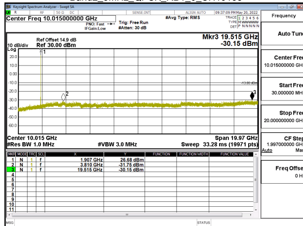
Band2_3MHz_QPSK_RB1_0_CH19185
