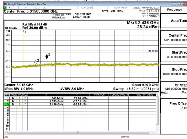
Band5_3MHz_QPSK_RB1_0_CH20635
