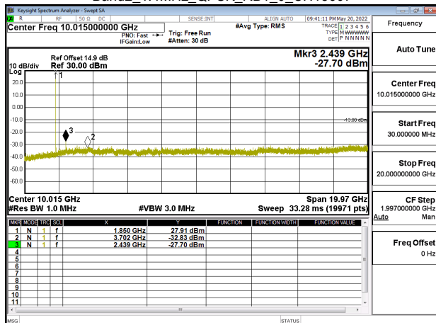
Band2_1.4MHz_QPSK_RB1_0_CH18900
