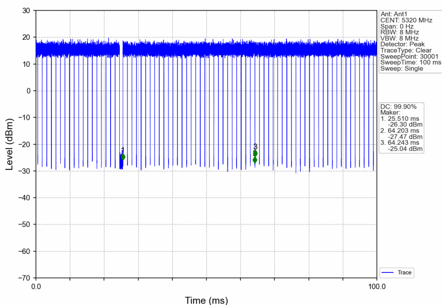
802.11n(HT20)_HCH_5320MHz_Ant1_NTNV
