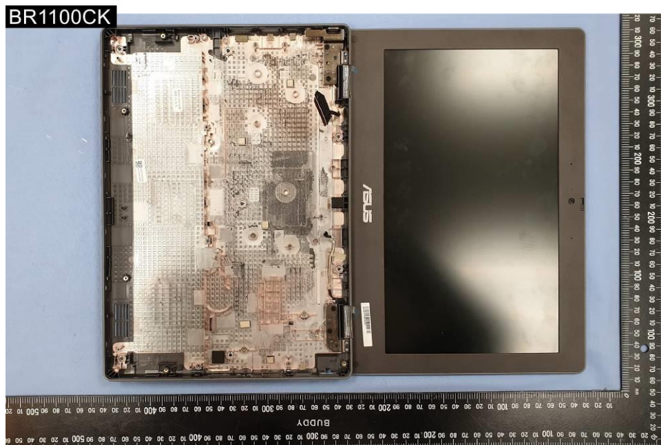
EUT Photo (14)
