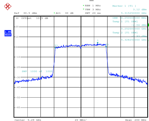
802.11ac80_5290MHz
