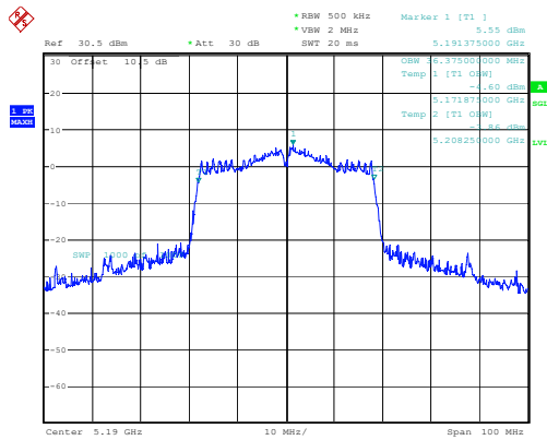
802.11ac40_5190MHz
