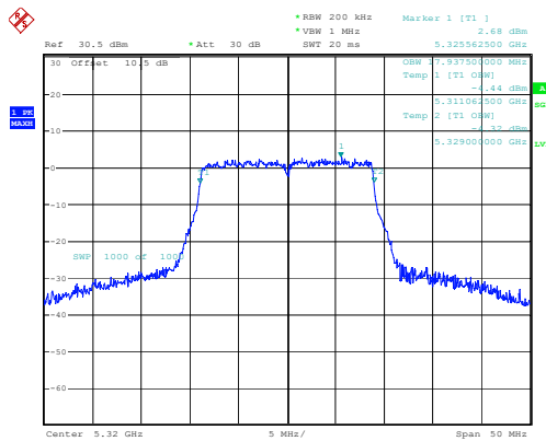
802.11ac20_5320MHz
