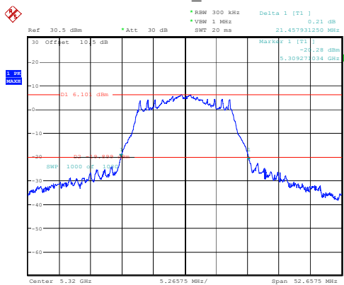
802.11a_5320MHz
