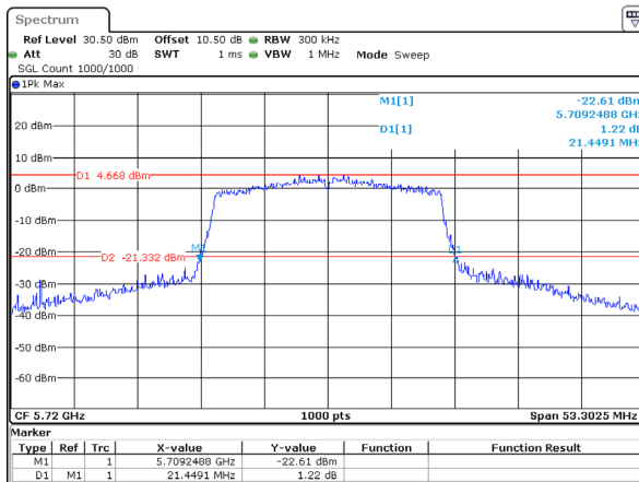
802.11ax20_5720MHz_RU_Full
