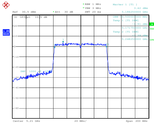
802.11ac80_5210MHz
