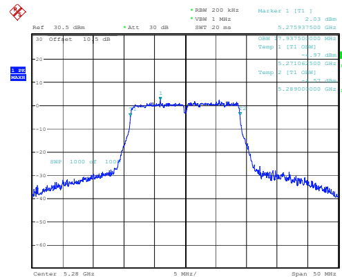
802.11ac20_5280MHz
