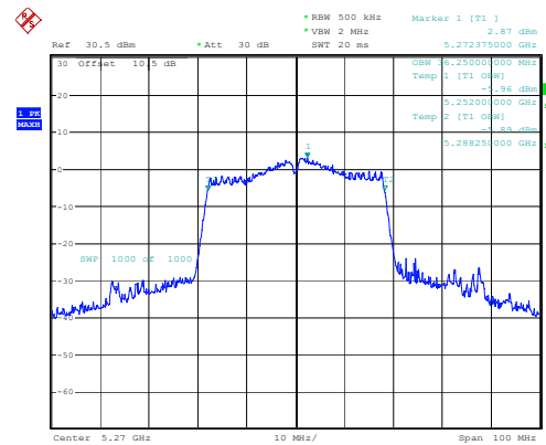
802.11ac40_5270MHz
