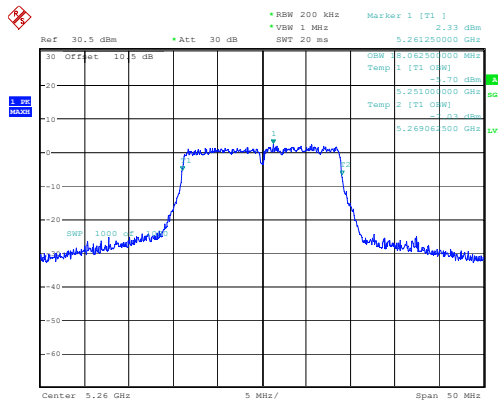
802.11ac20_5260MHz
