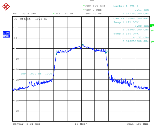
802.11ac40_5310MHz
