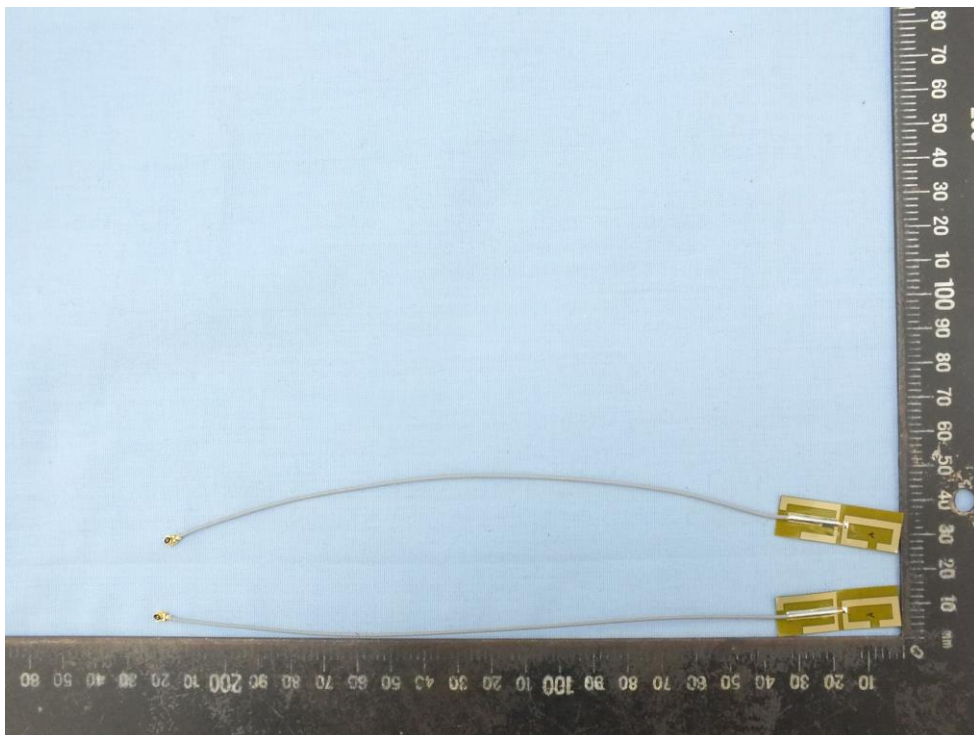
Antenna: Laird MAF95310 Mini NanoBlade Flex
