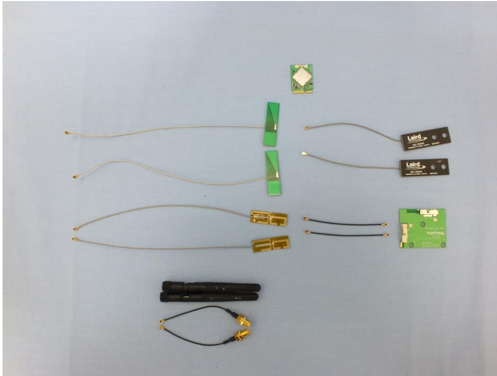
Antenna: Laird MAF94051
