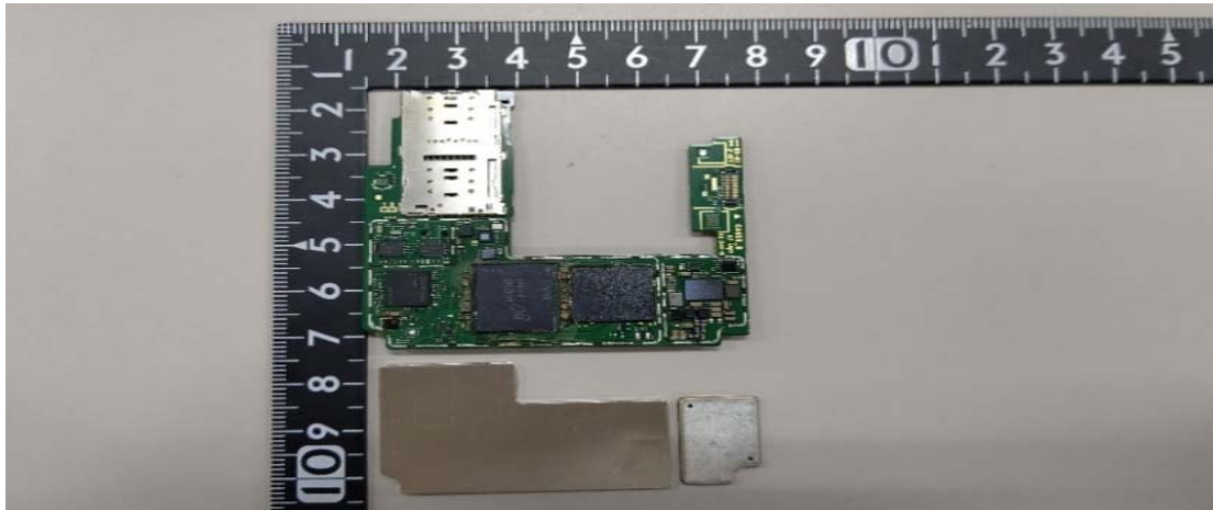
【IP PCB】
