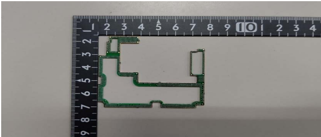
【IP PCB】
