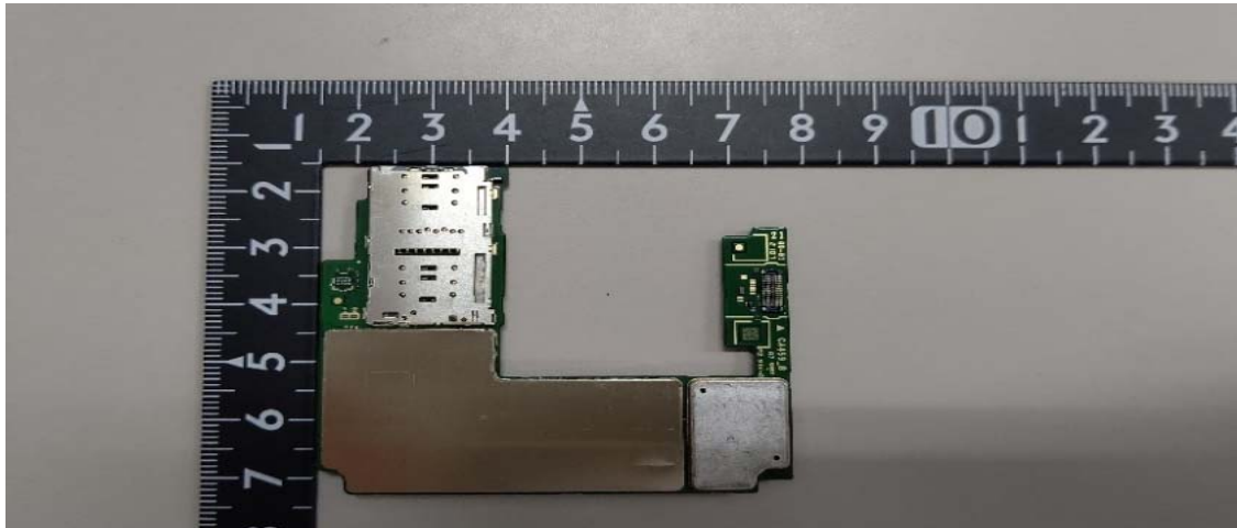
【BB PCB】
