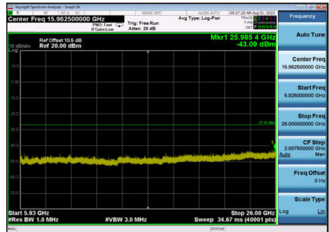
U-NII-3 ,Plot 3,5925MHz~26000MHz-802. 11ac(20MHz),5785MHz,Ant1
