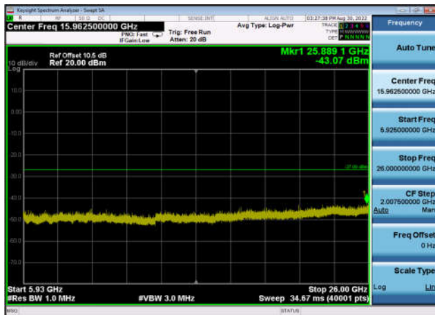
U-NII-3 ,Plot 3,5925MHz~26000MHz-802. 11ac(20MHz),5825MHz,Ant0
