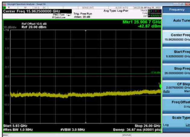
U-NII-3 ,Plot 3,5925MHz~26000MHz-802. 11a(20MHz),5785MHz,Ant0
