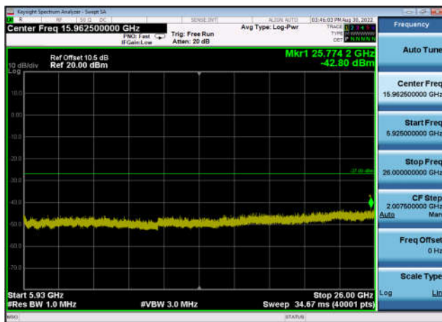
U-NII-3 ,Plot 3,5925MHz~26000MHz-802. 11ac(80MHz),5775MHz,Ant0
