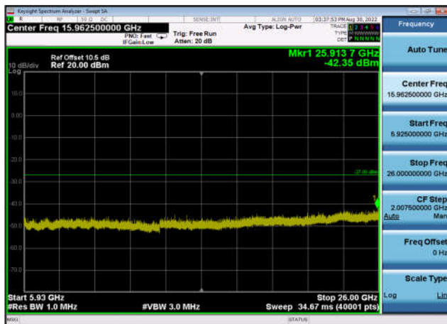
U-NII-3 ,Plot 3,5925MHz~26000MHz-802. 11ac(40MHz),5795MHz,Ant0
