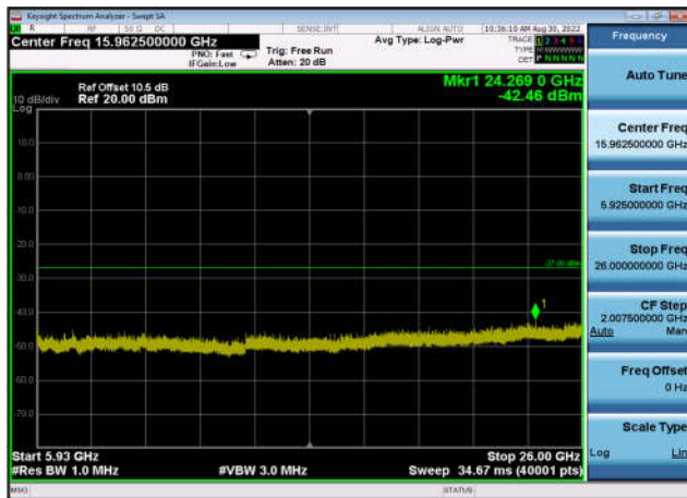
U-NII-3 ,Plot 3,5925MHz~26000MHz-802. 11a(20MHz),5825MHz,Ant0
