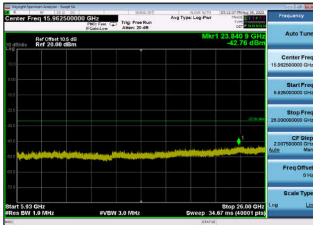
U-NII-3 ,Plot 3,5925MHz~26000MHz-802. 11ac(20MHz),5785MHz,Ant0
