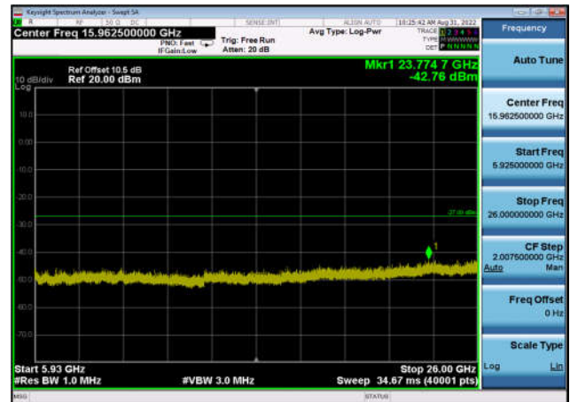
U-NII-3 ,Plot 3,5925MHz~26000MHz-802. 11ax(20MHz),5785MHz,Ant1
