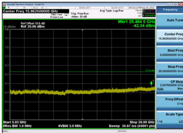
U-NII-3 ,Plot 3,5925MHz~26000MHz-802. 11ax(20MHz),5825MHz,Ant0
