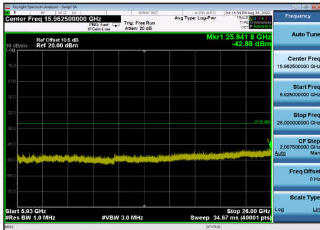
U-NII-3 ,Plot 3,5925MHz~26000MHz-802. 11ax(20MHz),5785MHz,Ant0
