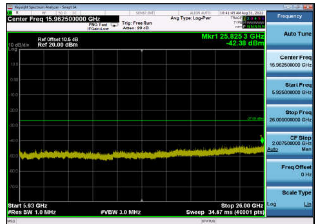
U-NII-3 ,Plot 3,5925MHz~26000MHz-802. 11ax(20MHz),5825MHz,Ant1
