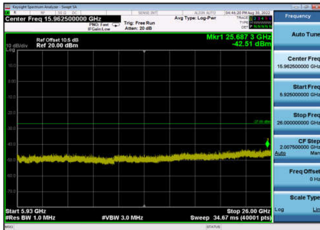
U-NII-3 ,Plot 3,5925MHz~26000MHz-802. 11ax(40MHz),5795MHz,Ant0
