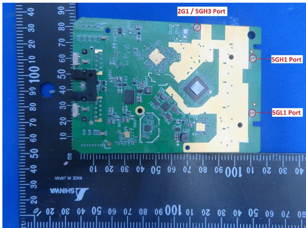
(24) EUT Photo
