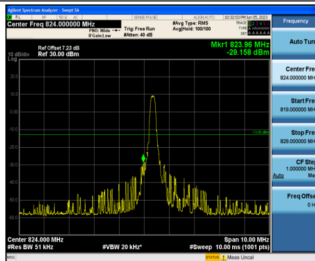
Band5-5MHz-QPSK-20425-1-0-Low--29.16-PASS
