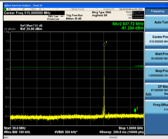
Band12-3MHz-16QAM-23165-1-0-Low-30-1000--61.23-PASS
