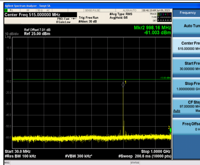
Band12-3MHz-16QAM-23095-1-0-Low-30-1000--61-PASS
