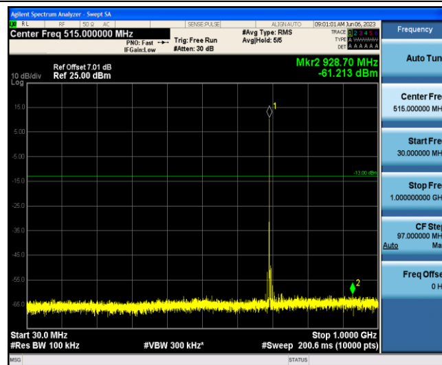
Band12-5MHz-QPSK-23035-1-0-Low-30-1000--61.21-PASS
