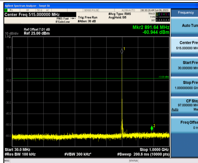
Band12-1.4MHz-QPSK-23095-1-0-Low-30-1000--60.94-PASS
