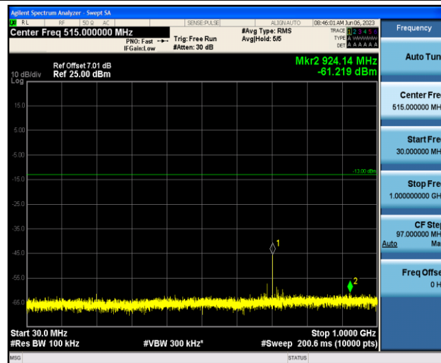
Band12-3MHz-QPSK-23095-1-0-Low-30-1000--61.22-PASS
