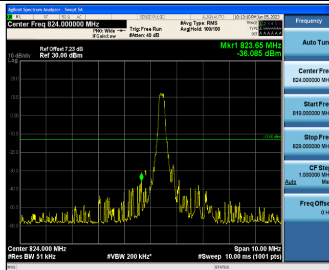
Band5-3MHz-QPSK-20415-1-0-Low--36.09-PASS
