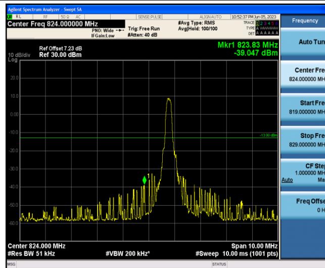
Band5-10MHz-QPSK-20450-1-0-Low--39.05-PASS
