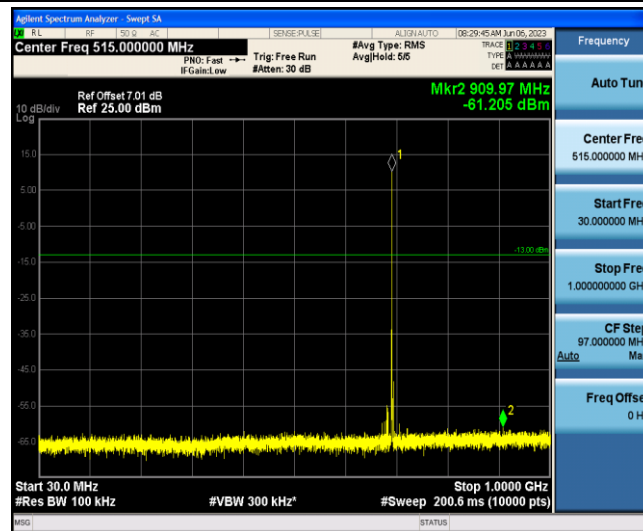
Band12-1.4MHz-QPSK-23017-1-0-Low-30-1000--61.21-PASS
