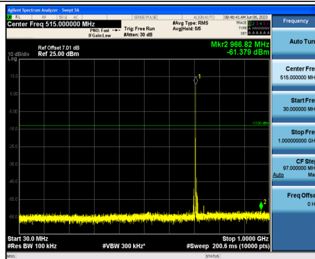
Band12-3MHz-QPSK-23165-1-0-Low-30-1000--61.38-PASS
