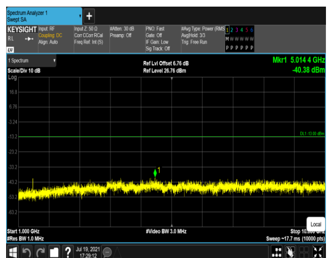
Band17-5MHz-QPSK-23825:1000~10000MHz
