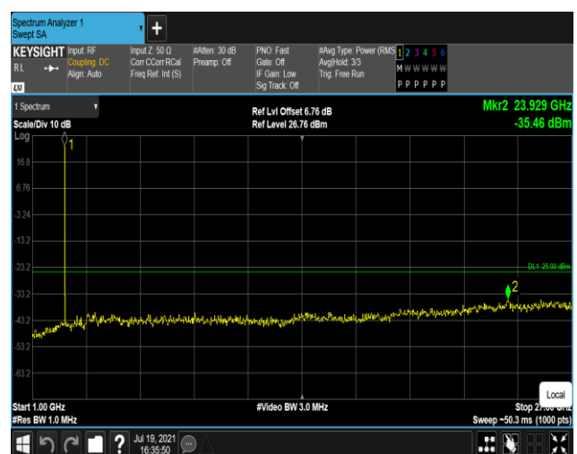
Band7-5MHz-QPSK-21425:1000~27000MHz
