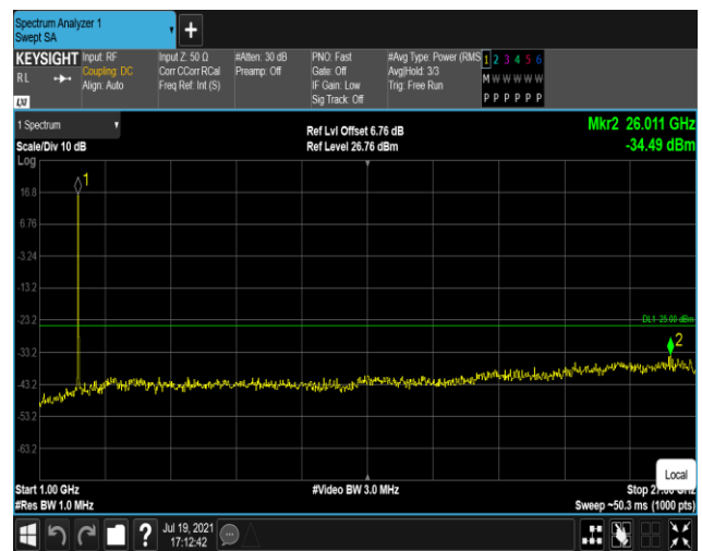
Band7-20MHz-16QAM-21350:1000~27000MHz
