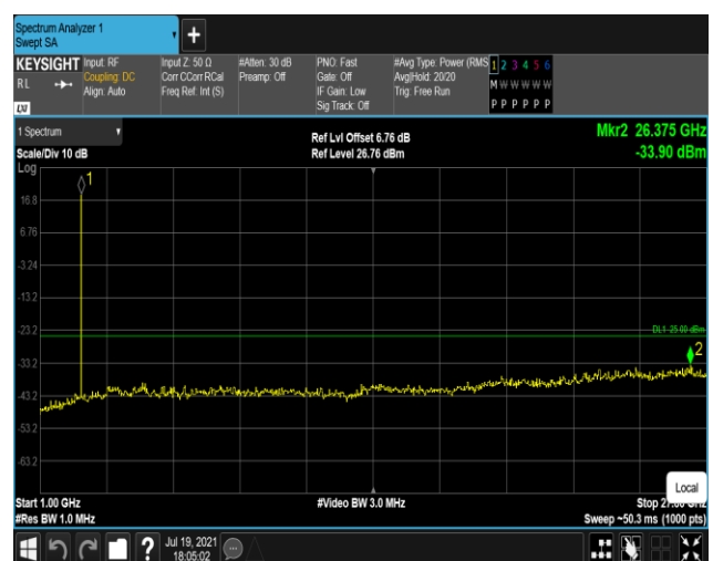
Band38-5MHz-QPSK-38225:1000~27000MHz
