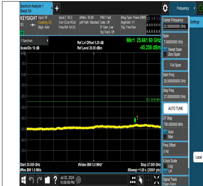
Band7-15MHz-QPSK-20825-1RB#0-20000~27000-PASS
