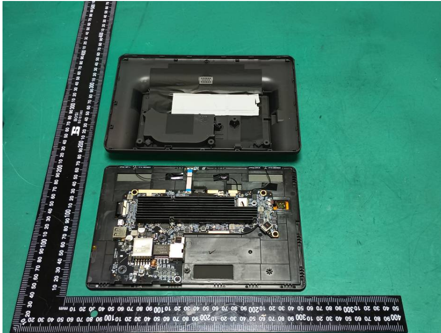
BLE ANT/Wi-Fi ANT1
