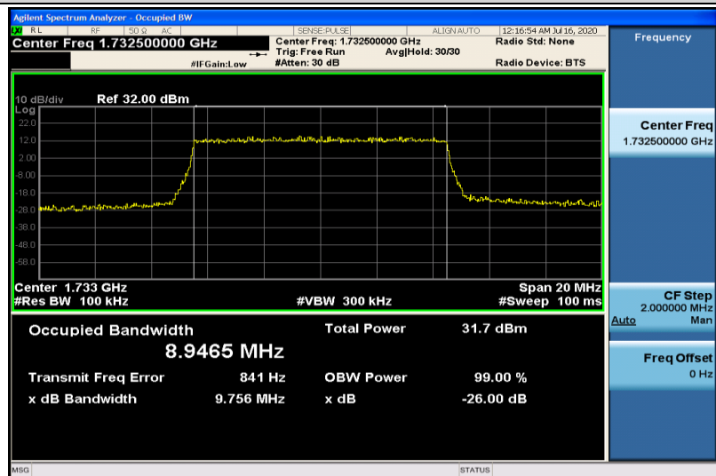
Band4-10MHz-QPSK-20175-50RB#0-8.9465
