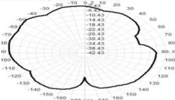
150.0MHz Total(E1-XZ), Max=-2.43dBi
