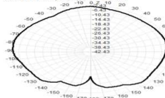
2450.0MHz Total(E2-YZ), Max=-3.08dBi
