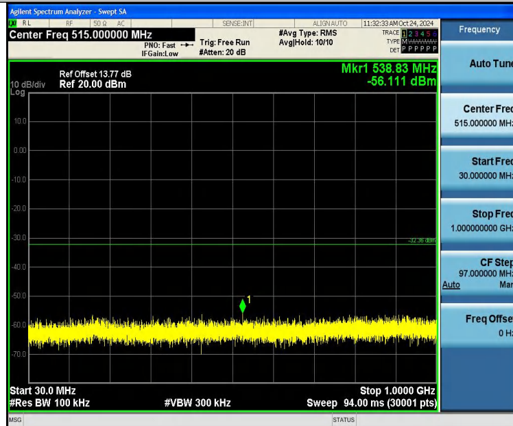
11G-Ant1-2437-30~1000-PASS
