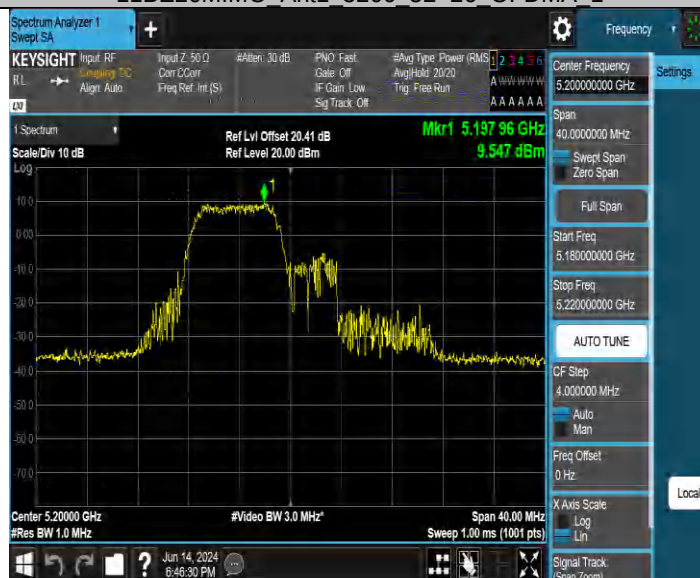
11BE20MIMO Ant2 5200 52+26 OFDMA 1
