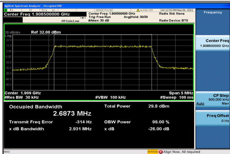
Band2-3MHz-QPSK-19185-15RB#0-2.6873
