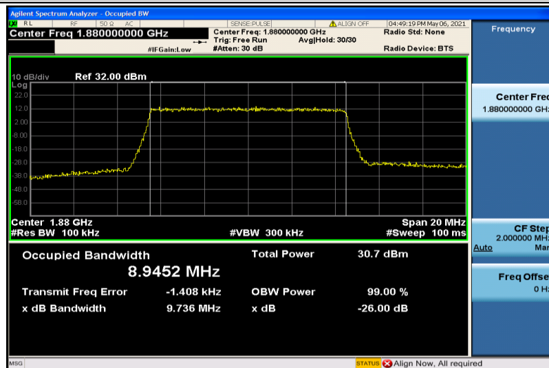
Band2-10MHz-QPSK-18900-50RB#0-8.9452
