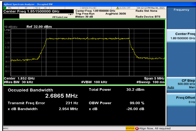
Band2-3MHz-QPSK-18615-15RB#0-2.6865
