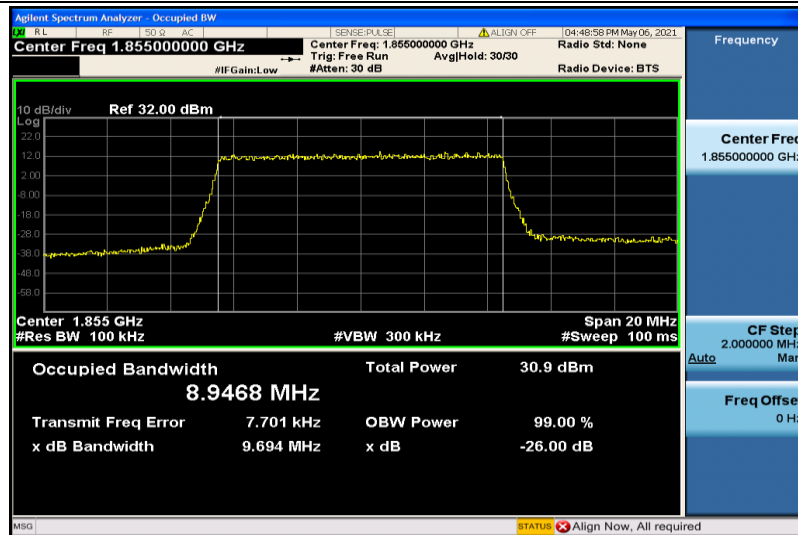
Band2-10MHz-QPSK-18650-50RB#0-8.9468
