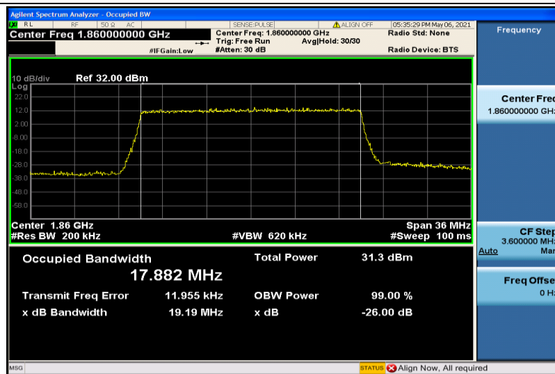
Band2-20MHz-QPSK-18700-100RB#0-17.882
