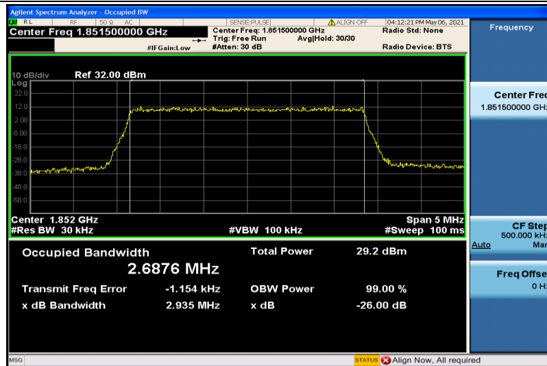
Band2-3MHz-16QAM-18615-15RB#0-2.6876
