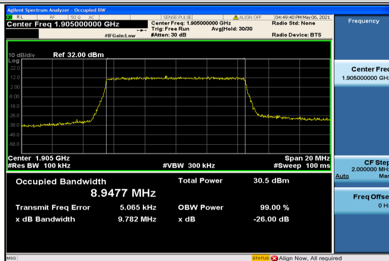
Band2-10MHz-QPSK-19150-50RB#0-8.9477
