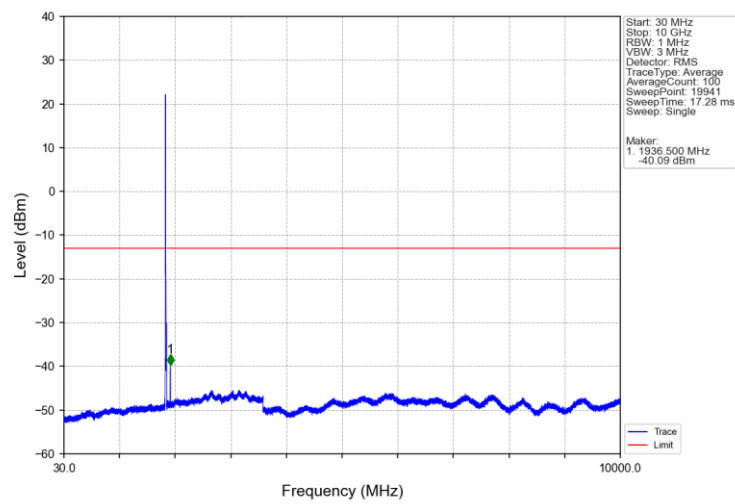
Band2_10MHz_16QAM_LCH_1855MHz_RB_1_0_NTNV
