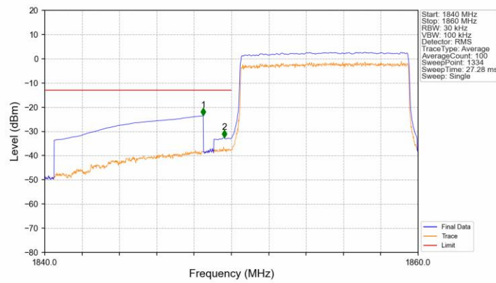
Band2_10MHz_16QAM_LCH_1855MHz_RB_50_0_NTNV
