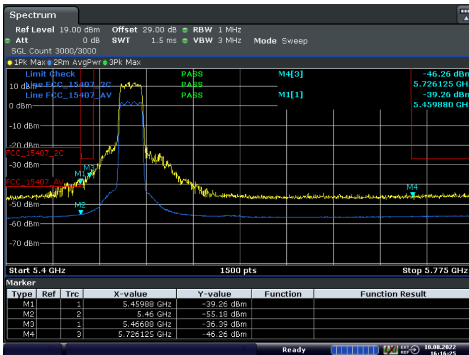
Antenna A
