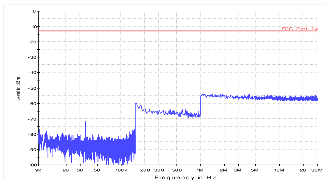
Fula2_FCC_24_Scan1_9kHz_30MHz
