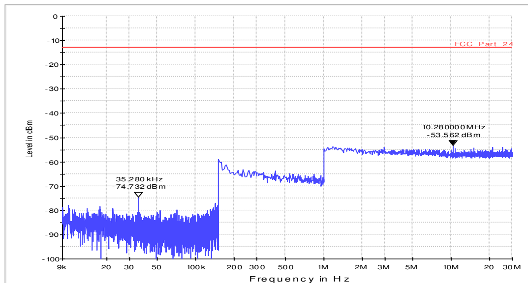
Fula2_FCC_24_Scan1_9kHz_30MHz
